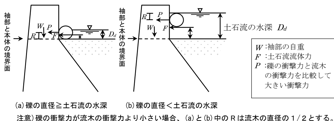
図－8 袖部の断面
