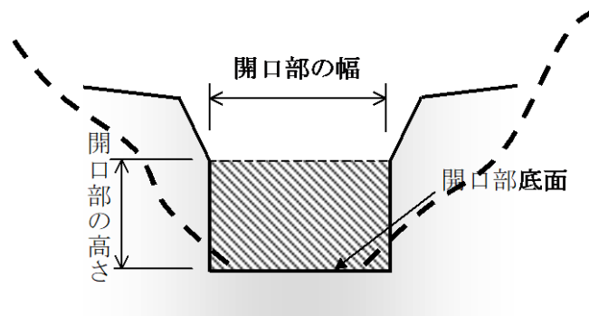
図－１４ 透過型砂防堰堤の開口部（斜線部）
