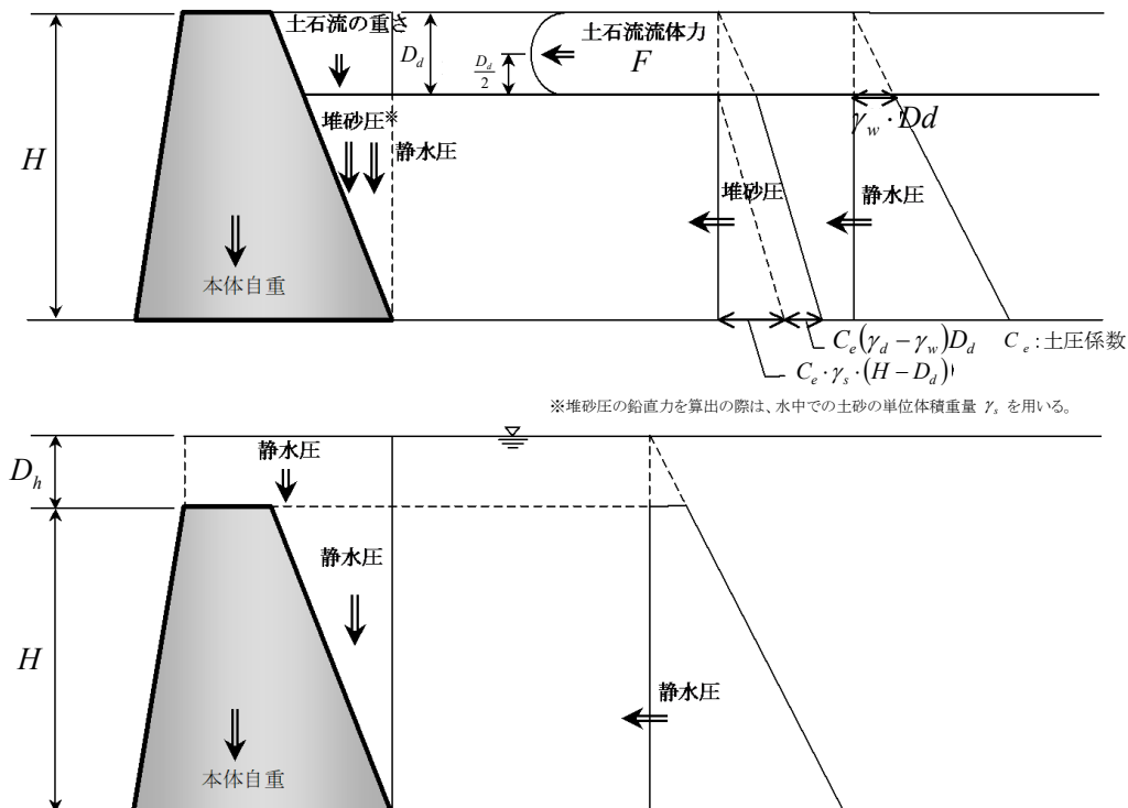
図－３ 不透過型砂防堰堤 越流部の設計外力図 ( H < 15\text{m} 、上段：土石流時、下段：洪水時)
