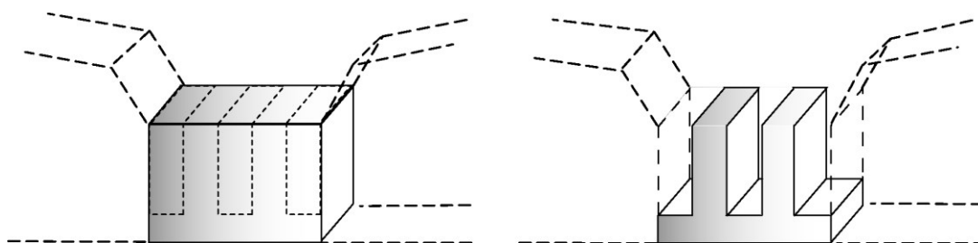
図－１１ スリット部における水通しの堤体積
