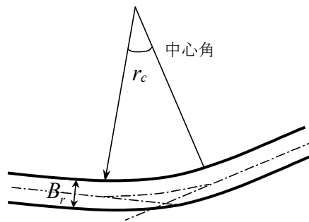
図－19 土石流導流工湾曲部の法線形
