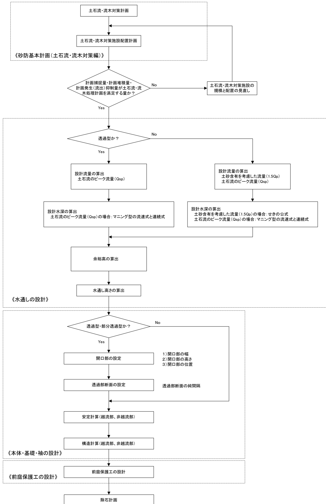
図ー２ 土石流・流木捕捉工設計の流れ
