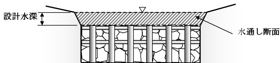
図－１３ 水通し断面（斜線部）
