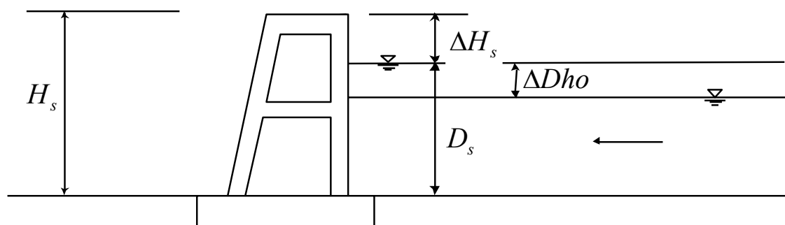
図一参 3 土砂礫等による閉塞の恐れのない場合の透過部の高さ
