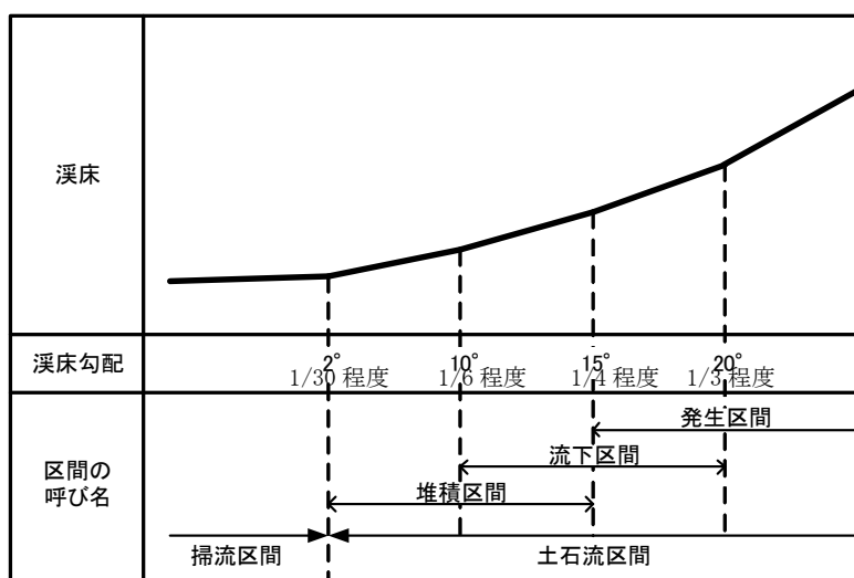
図－1 土砂移動の形態の溪床勾配による目安 1)
