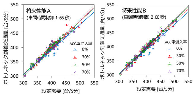
図 6 ACC 車混入率ごとのボトルネック到着交通量の比較
