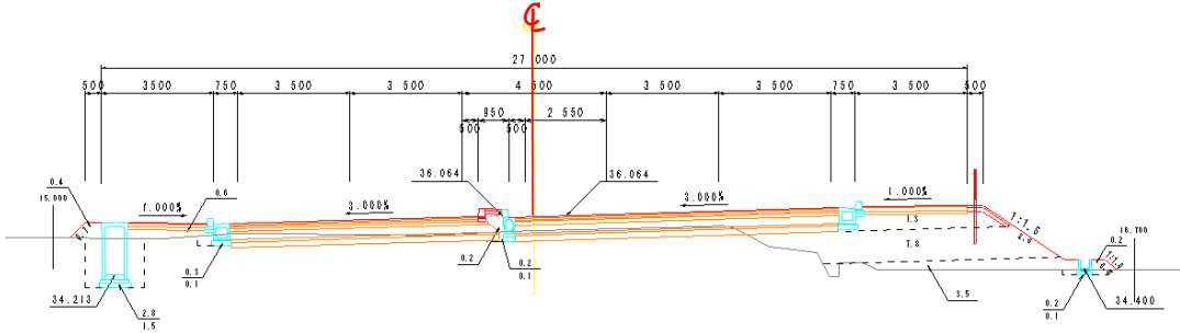
図 2-7 サンプルとなる横断図
