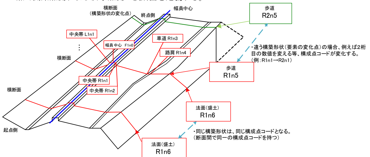
図 4-18 構成点コードの考え方（コード番号は例）
