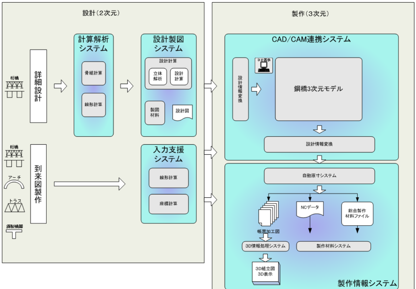
図 - 2 CAD/CAM システムの概要
