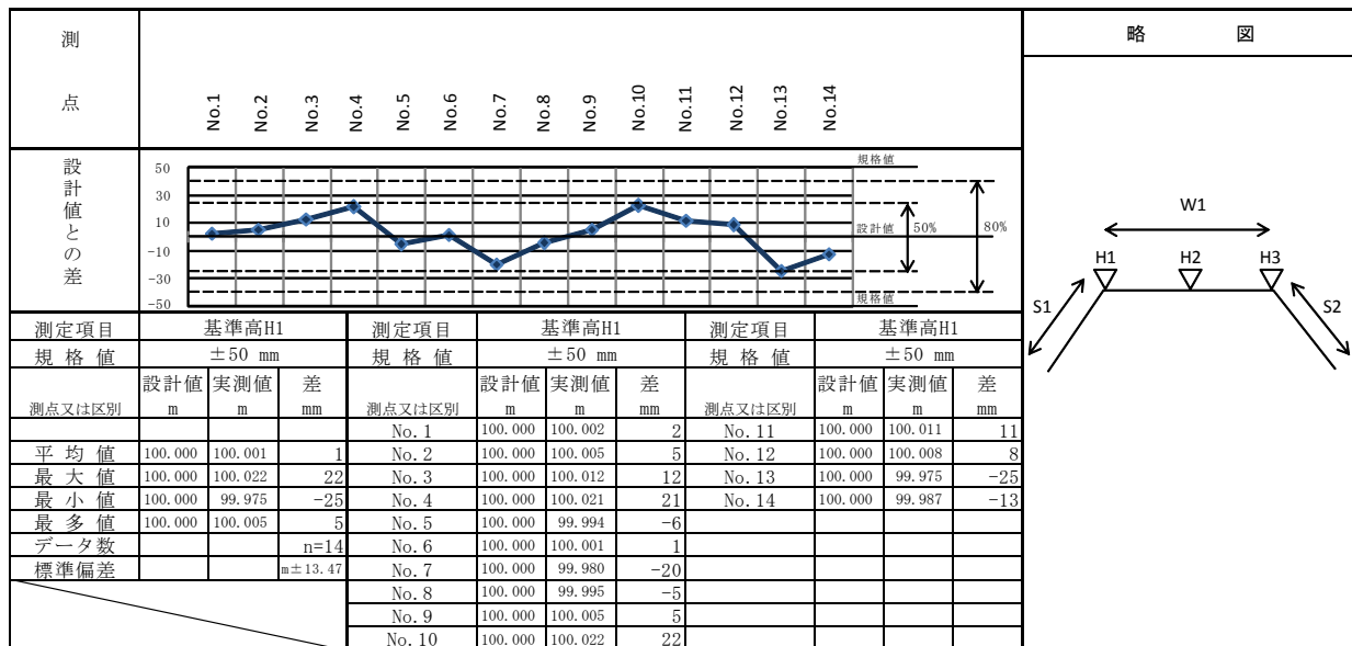
図 1-11 出来形管理図表 作成例
