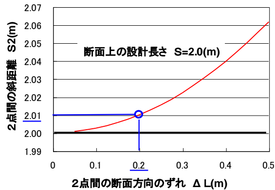
図 2-1 管理断面上の出来形計測点誤差が及ぼす長さ誤差の影響範囲
