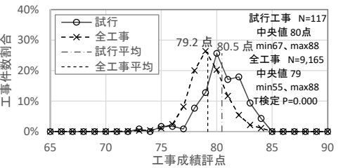
図-4 チャレンジ型の工事品質（9整備局）
