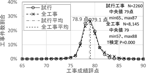
図-5 地元企業活用型の工事品質（4整備局）
