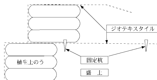
図B 巻込み工法(植生土のう)参考図
