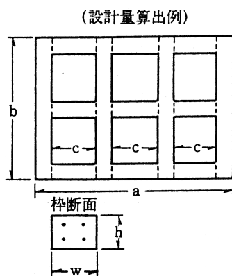
(4本配筋の例)
