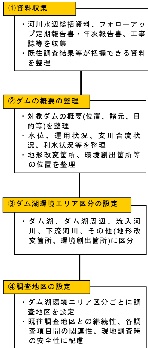
図 5-11 調査地区の設定フロー【ダム湖版】
