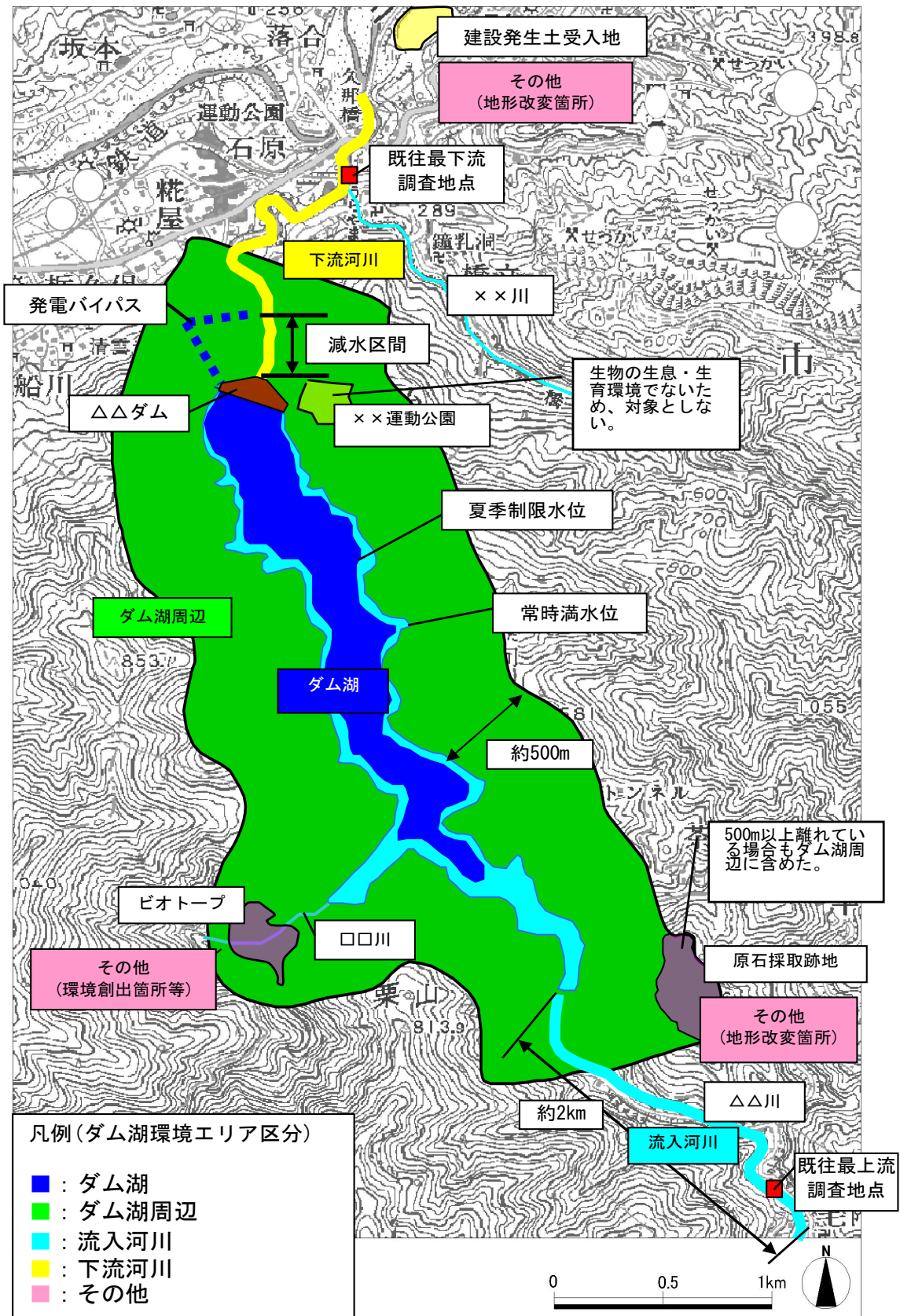
図 5-13 ダム湖環境エリア区分図(例)
