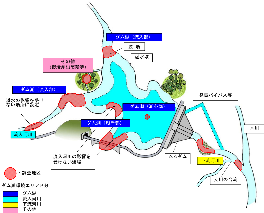
図 5-17 調査地区の配置例(底生動物調査)
