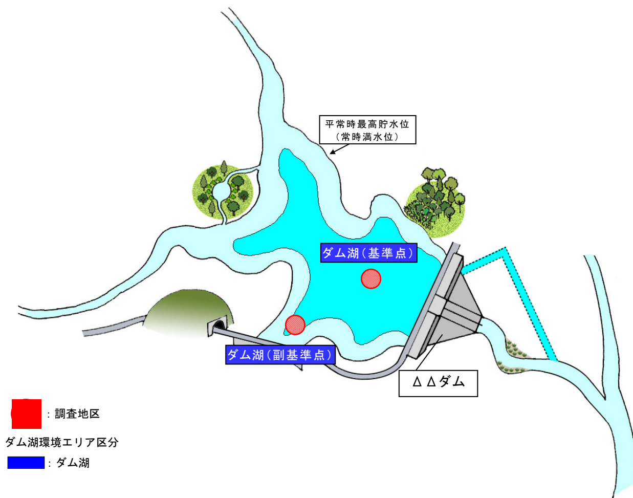
図 5- 18 調査地区の配置例(動植物プランクトン調査)
