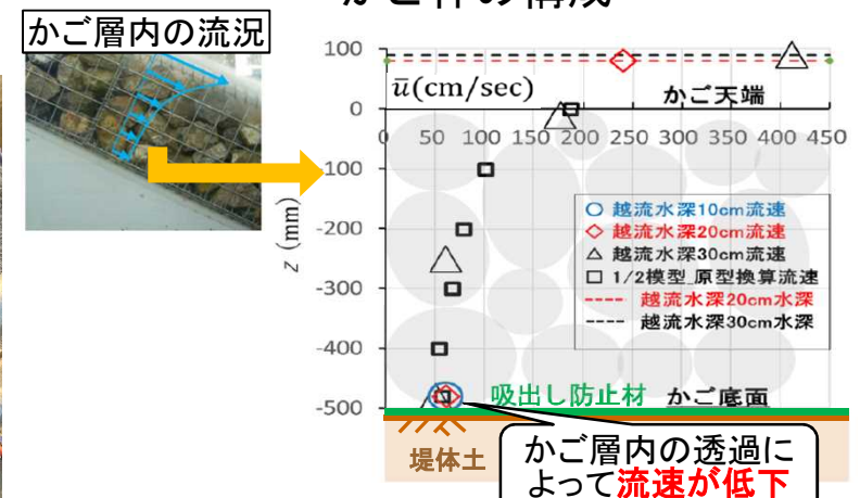
かご層内外の流速垂直分布 (文献 1) に一部加筆)
