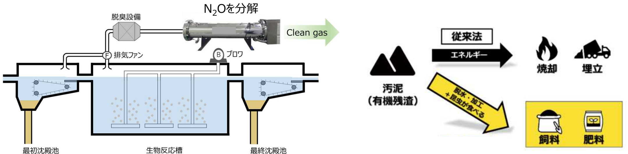
① 紫外光を用いた N_2O , CH_4 の分解技術による水処理からの温室効果ガス排出抑制
