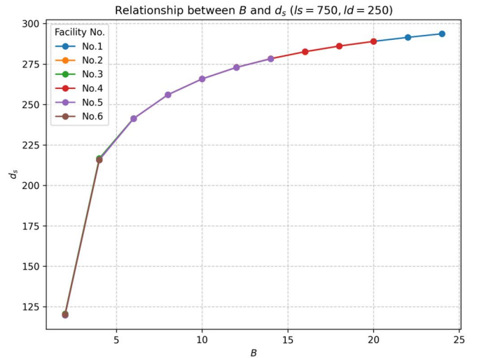
図-C.12 d_s - B グラフの結果 ( l_s=750\text{mm} , l_d=250\text{mm} )
