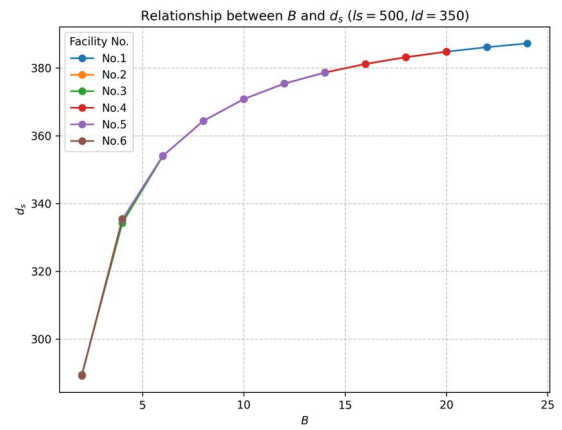
図-C. 52 d_s - B グラフの結果 ( l_s=500\text{mm} , l_d=350\text{mm} )
