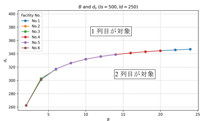
図4.6 B-d_{slim} グラフ ( c_l=200\text{mm} ， l_s=500\text{mm} ， l_d=250\text{mm} )
