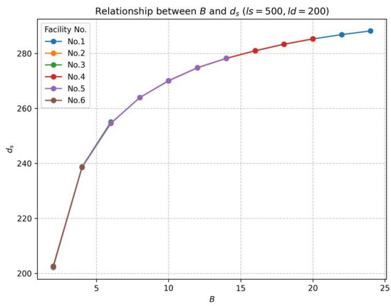
図-C. 49 d_s - B グラフの結果 ( l_s=500\text{mm} , l_d=200\text{mm} )
