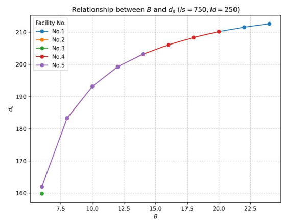
図-C. 54 d_s - B グラフの結果 ( l_s=750\text{mm} , l_d=250\text{mm} )
