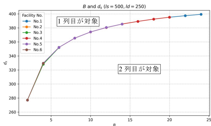
図4.4 B-d_{slim} グラフ ( c_l=400\text{mm} ， l_s=500\text{mm} ， l_d=250\text{mm} )
