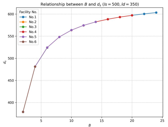
図-C.10 d_s - B グラフの結果 ( l_s=500\text{mm} , l_d=350\text{mm} )
