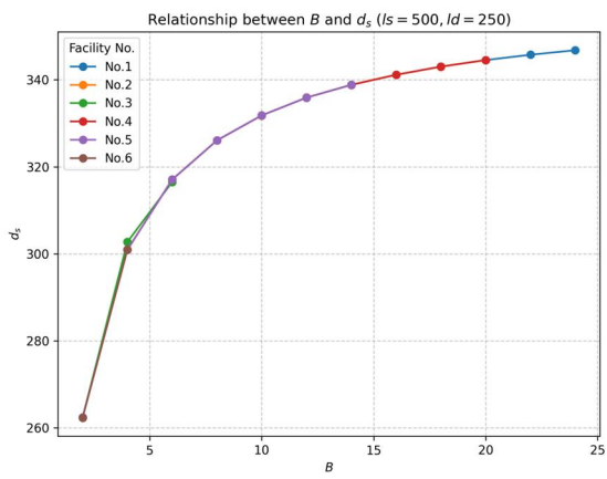
図-C. 50 d_s - B グラフの結果 ( l_s=500\text{mm} , l_d=250\text{mm} )
