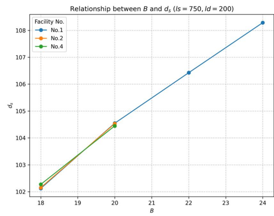
図-C. 53 d_s - B グラフの結果 ( l_s=750\text{mm} , l_d=200\text{mm} )
