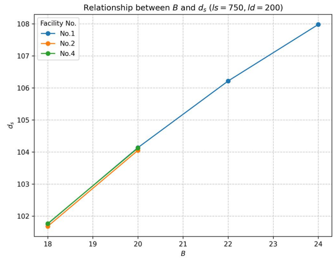
図-C.11 d_s - B グラフの結果 ( l_s=750\text{mm} , l_d=200\text{mm} )
