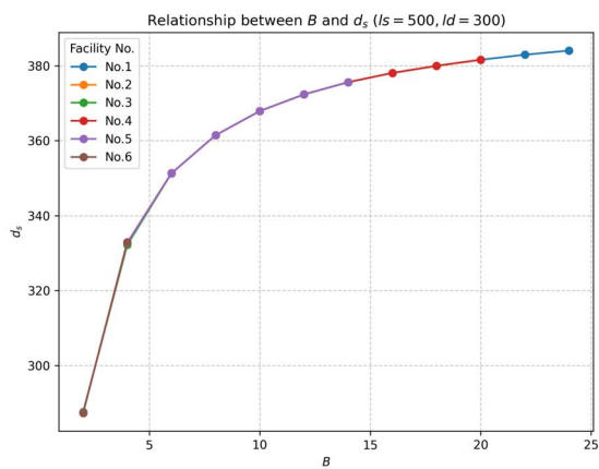
図-C. 51 d_s - B グラフの結果 ( l_s=500\text{mm} , l_d=300\text{mm} )
