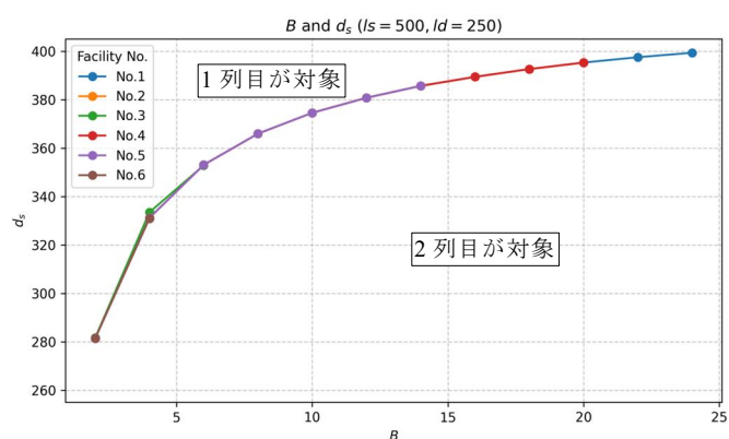
図4.5 B-d_{slim} グラフ ( c_l=300\text{mm} ， l_s=500\text{mm} ， l_d=250\text{mm} )
