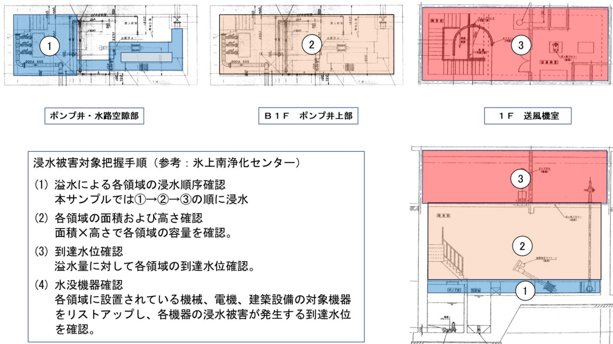
図2-6-16 氷上南浄化センター 浸水順
