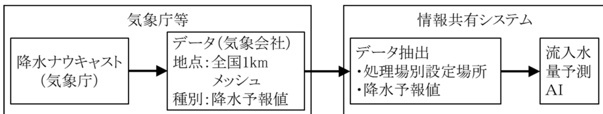
図2-2-1 降水量予報値のデータ取得フロー
