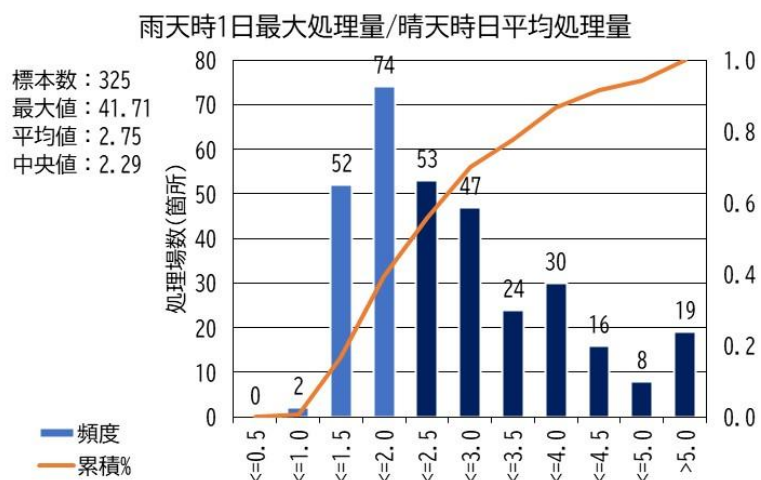
図2-7-6 雨天時1日最大汚水量/晴天時日平均処理量別の処理場数
