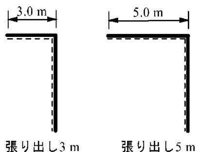
図－4.1.5 張り出し型遮音壁の例
