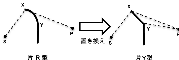
図－4.1.6 片R型遮音壁の片Y型への置換例
