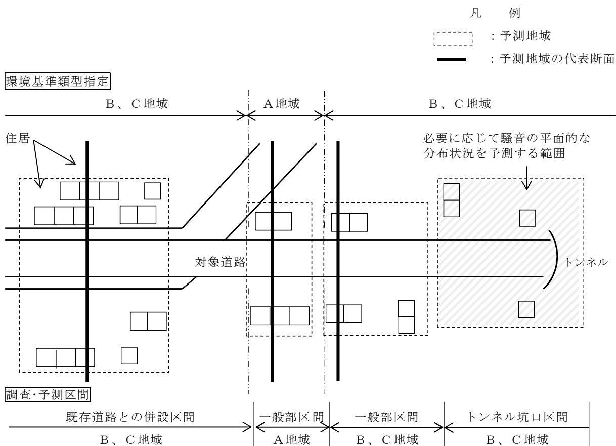
図－4.1.4 予測地域の代表断面の設定例
