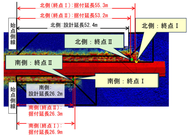
図-A.17 TIN 法出来形(石垣港 UAV グリーンレーザ測量)
