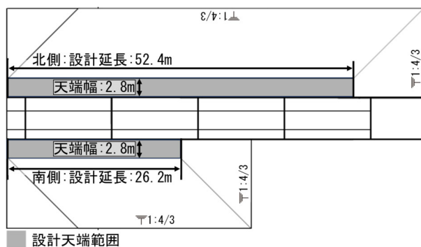
図-A.6 石垣港設計図面
