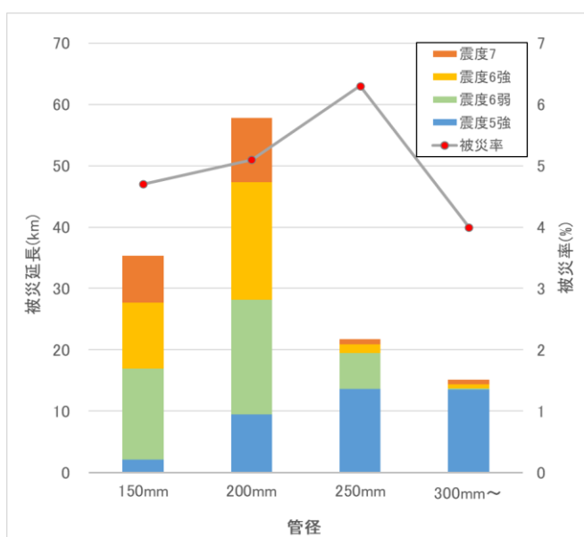
図4 塩ビ管の管径別の被災率
