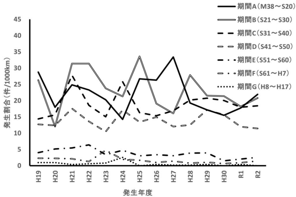
図4 発生年度、布設期間別発生割合 (CP)
