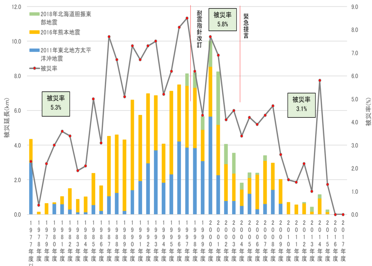
図 1 布設年度別の被災率
