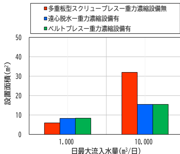
図 2 OD 法における汚泥脱水機の設置面積
