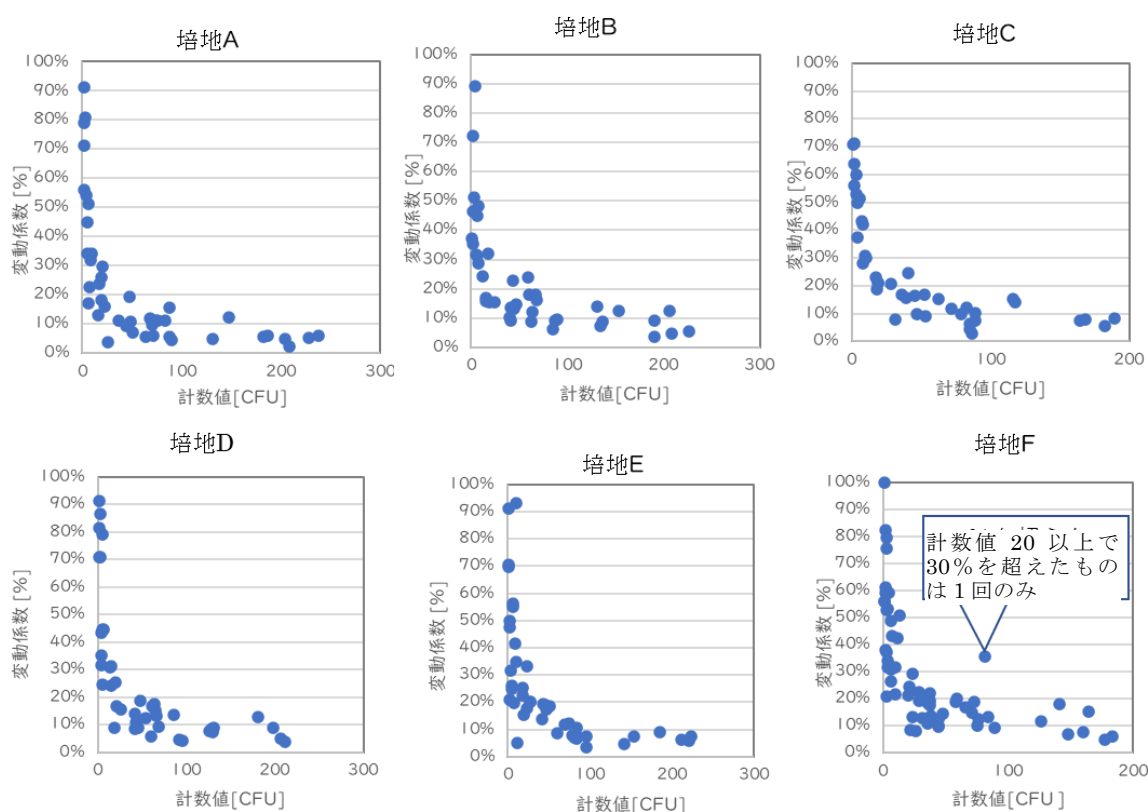
図4 2021 年の特定酵素培地による大腸菌数測定結果に基づく計数値と変動係数
