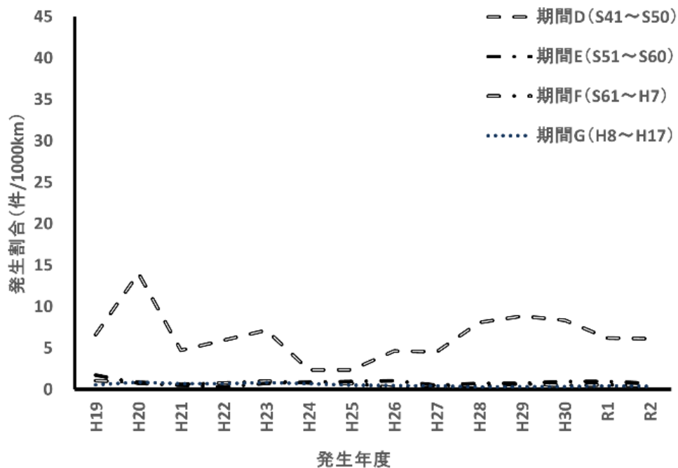
図5 発生年度、布設期間別発生割合 (VU)
