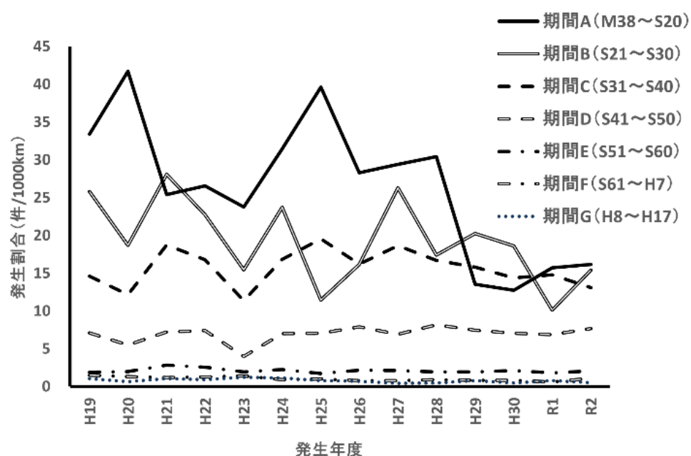
図3 発生年度、布設期間別発生割合（HP）
