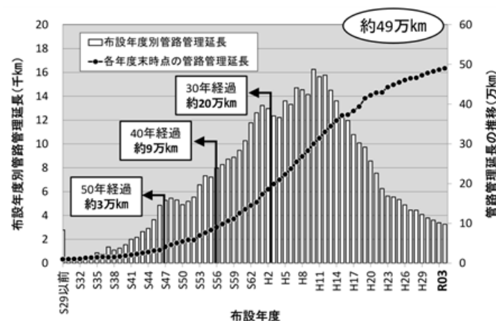
図1 管路管理延長と老朽管延長
