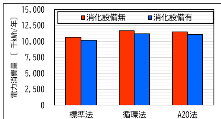
遠心濃縮—スクリープレス脱水
