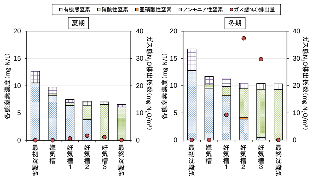
図 1 系列②における夏期と冬期の槽ごとの \text{N}_2\text{O} 排出係数と各態窒素濃度 4)
