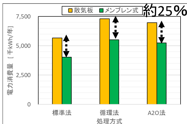
図 3 標準法、循環法、A 2 O 法における散気装置別の水処理設備の電力消費量
