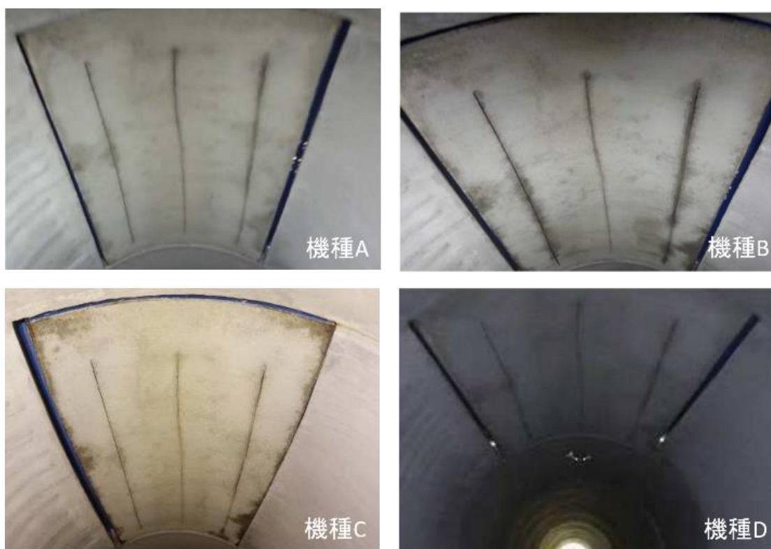
図9 ドローン調査機器の機種別の模擬異常の撮影写真（クラック（軸方向））
