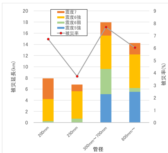
図3 コンクリート管の管径別の被災率
