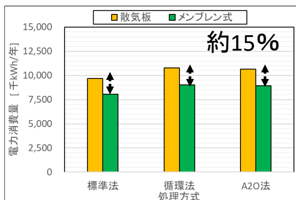
図 4 標準法、循環法、A 2 O 法における散気装置別の水処理設備・汚泥処理設備の電力消費量
