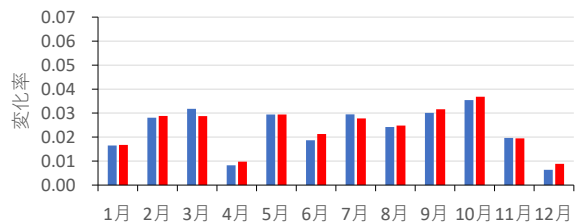
図5-3 月平均最低気温の変化率
