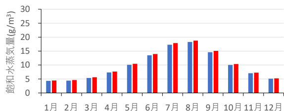
図 6-3 月平均最低飽和水蒸気量
