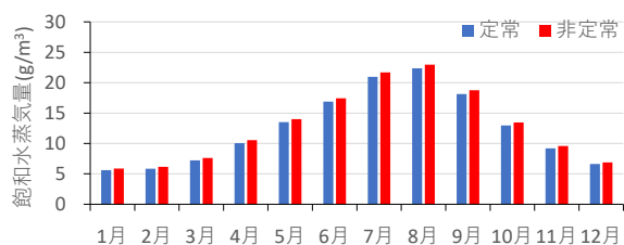
図 6-1 月平均飽和水蒸気量
