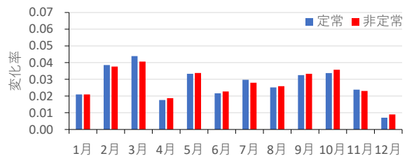
図5-1 月平均気温の変化率
