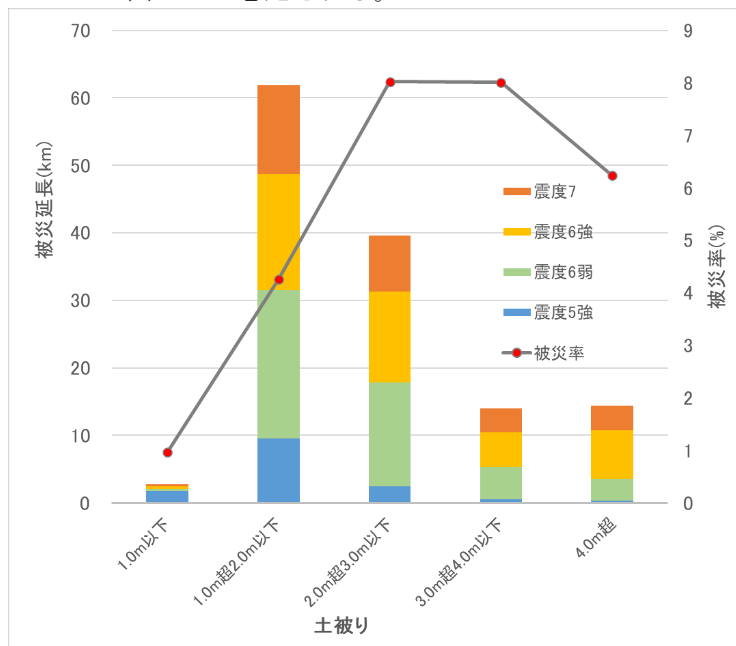
図 2 土被り別の被災率
