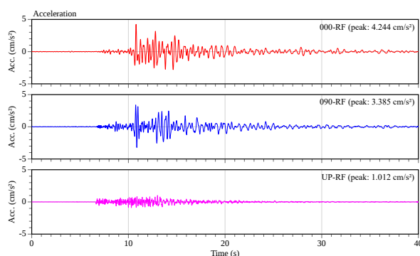
(ii) 屋上加速度波形 (WJMC4)
