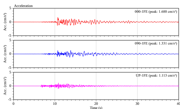
(i) 1 階加速度波形 (WJMC2)
