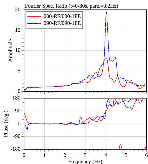
(iv) フーリエスペクトル比
