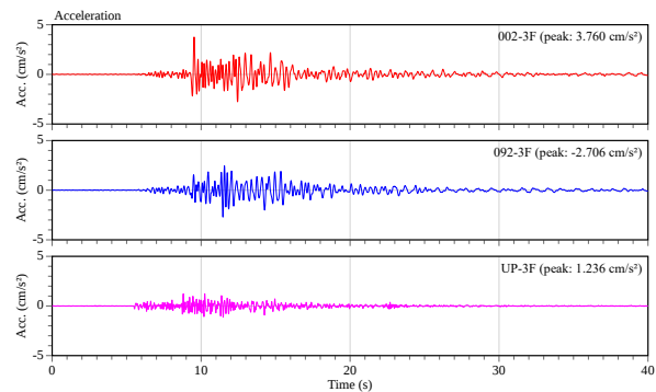
(ii) 3 階加速度波形_北側 (WJMF4)
