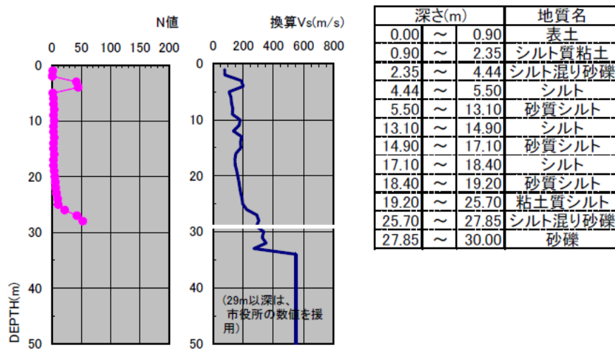
図 4.5-3 輪島市役所の土質図 4.5-3)
