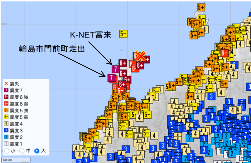
図 4.1-1 令和 6 年能登半島地震の震度分布図 4.1-3)
