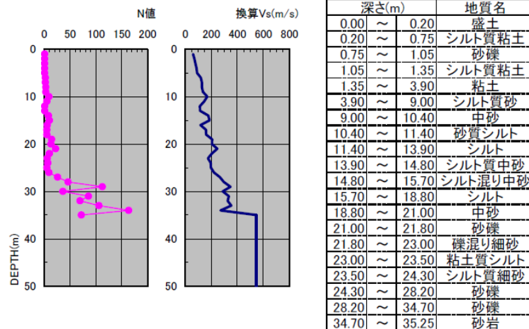
図 4.5-2 気象庁輪島 (WJMC) の土質図 4.5-3)
