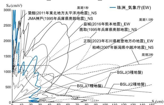
S_a-S_d 曲線
