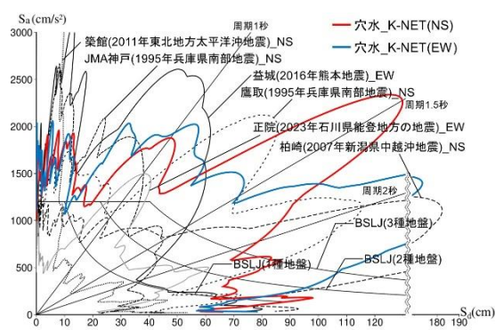
S_a-S_d 曲線
