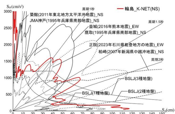
S_a-S_d 曲線
