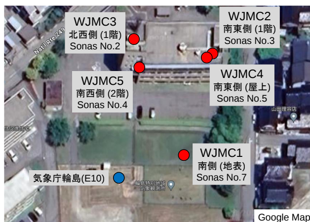
図 4.4-3 WJMC 強震計設置位置
