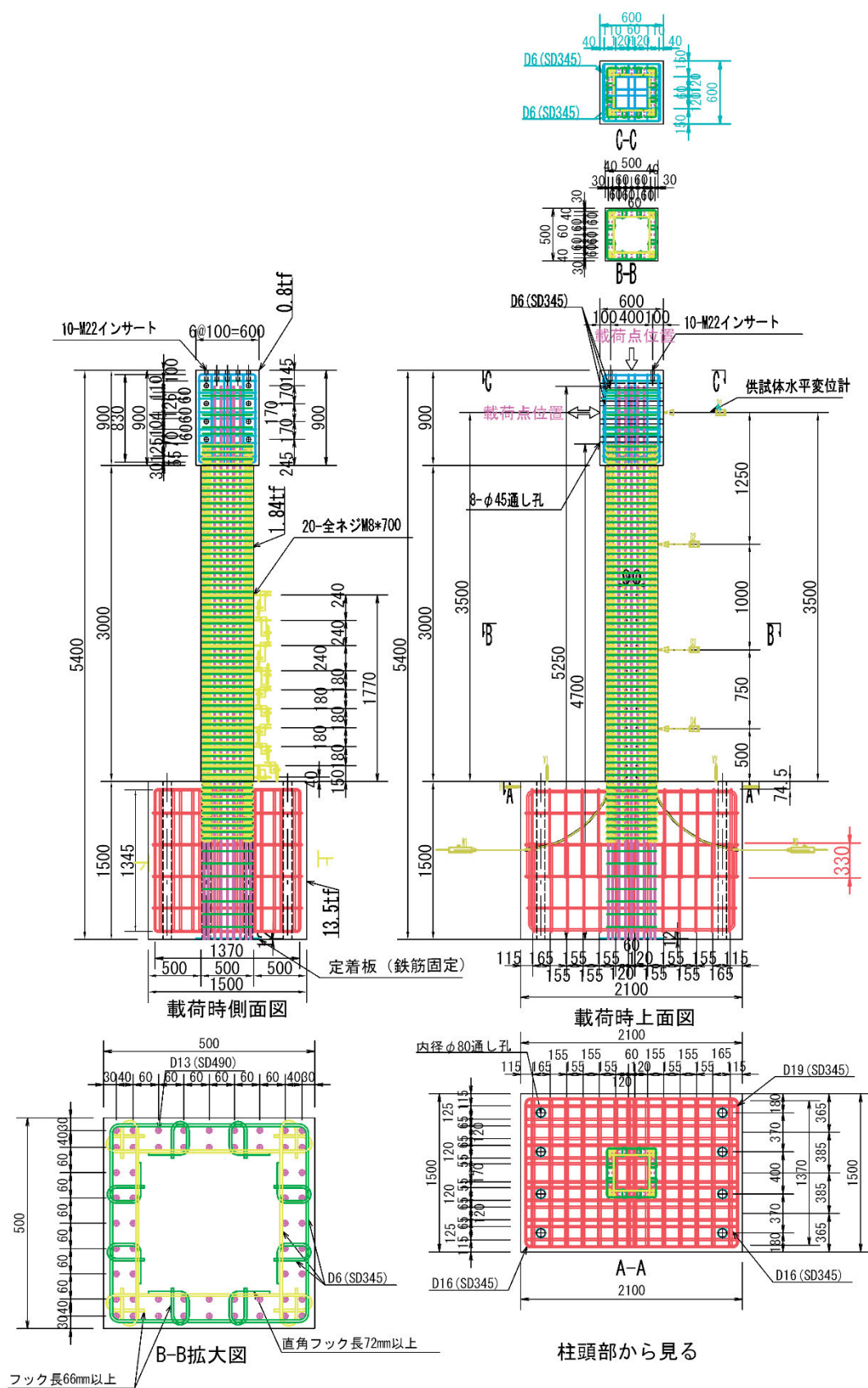
付図 4.2.5 シリーズ D2-1, D2-2 供試体配筋図
