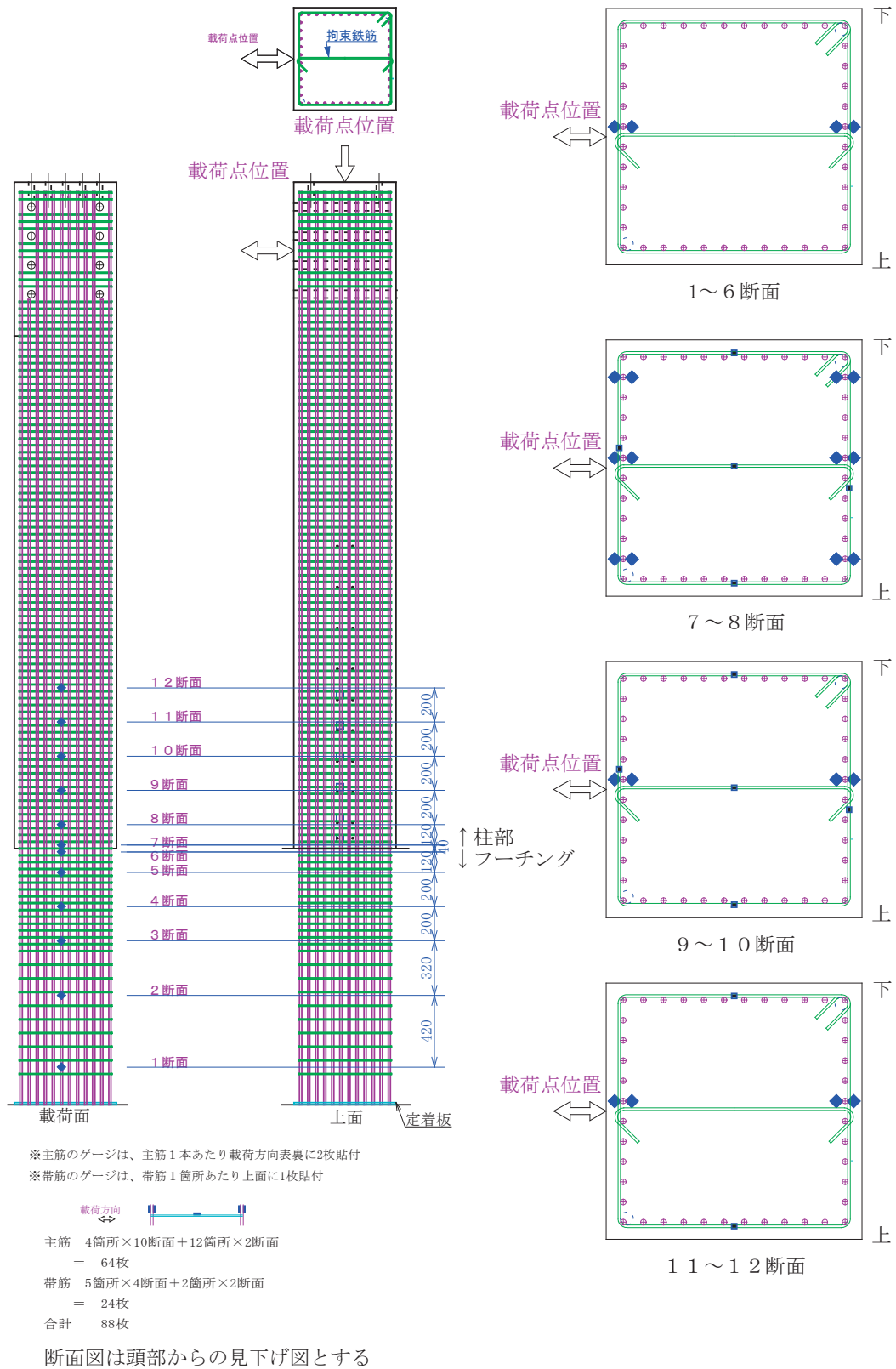
付図 4.2.10 シリーズ D1-3 ひずみゲージ位置及び数量図
