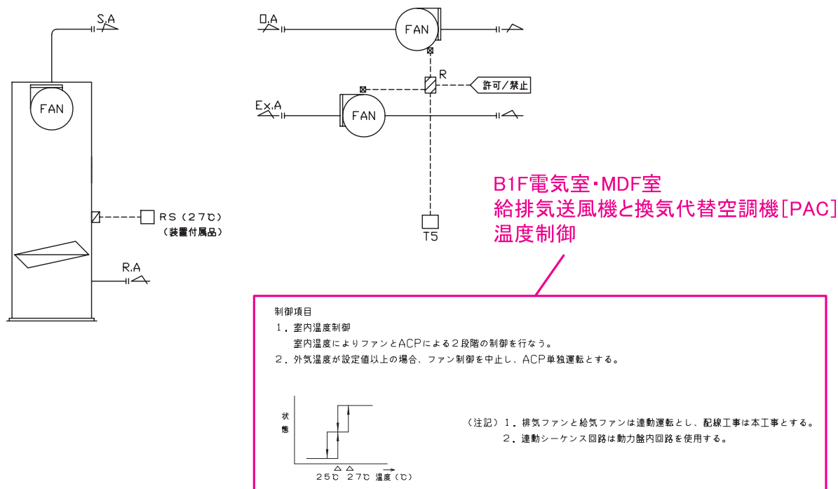
図 3-3-7 空調設備自動制御フロー図 (7) (図面 - 空 -24 : 換気設備部分を抜粋)
