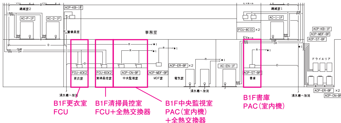
図 3-2-34* 空調設備配管系統図 (図面 - 空 - 16 : 地下 1 階部分を抜粋)
