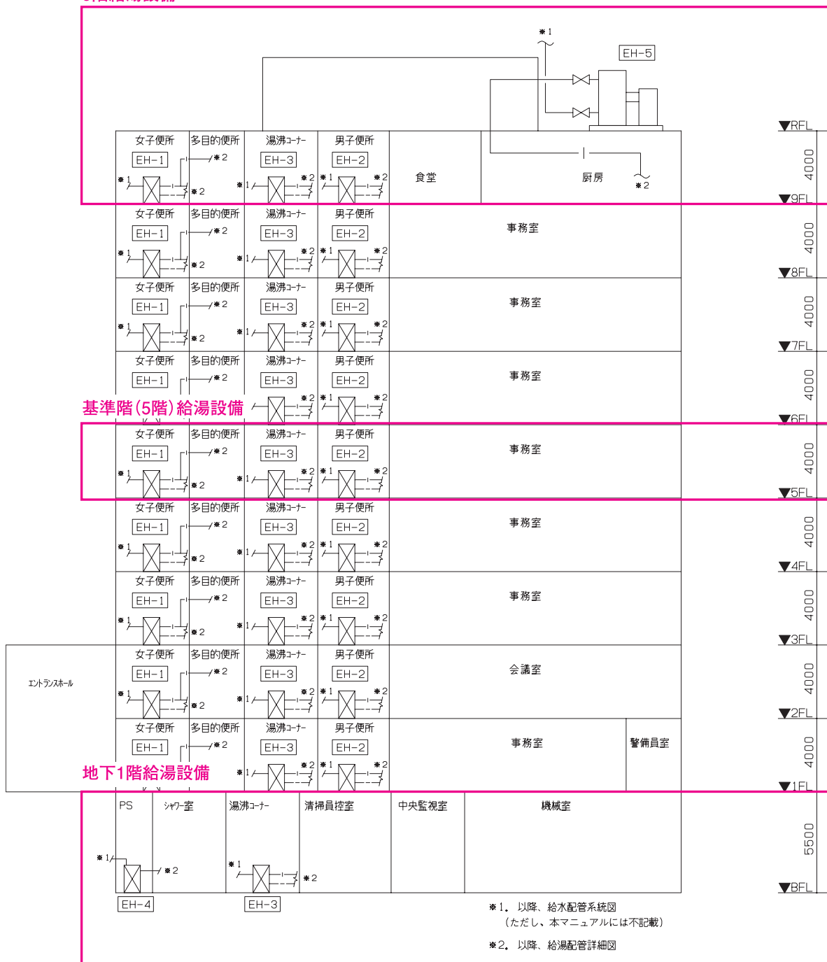
図 3-5-4* 衛生設備配管系統図 (図面 - 衛 -2)
