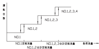
図 3-2-23 空調設備自動制御フロー図 (1) (図面 - 空 - 18)
