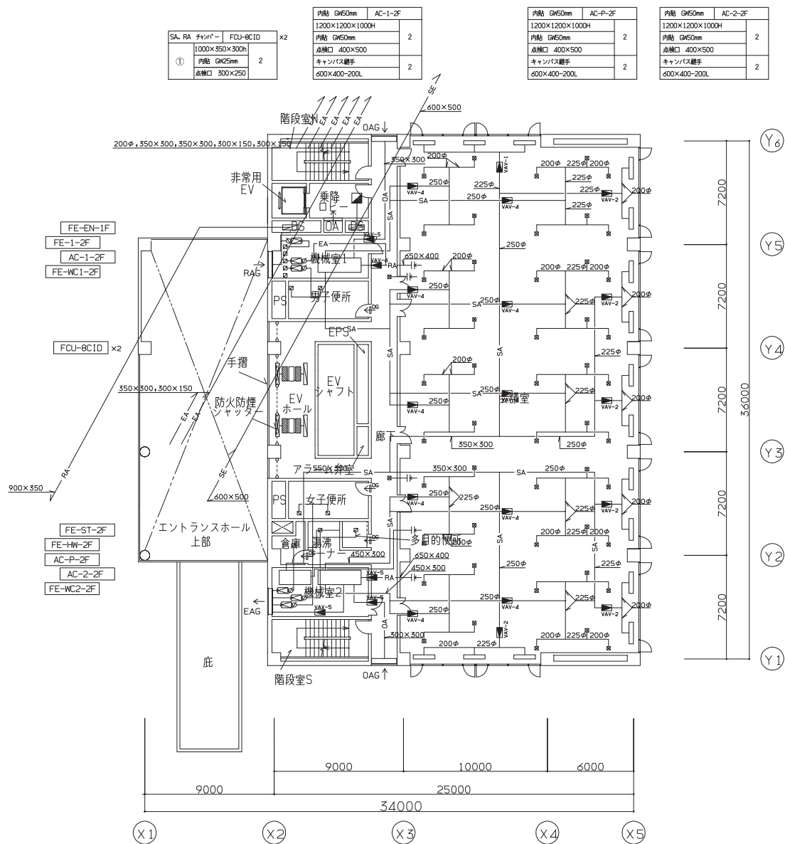
図面一空一 12 空調設備 2 階ダクト平面図
