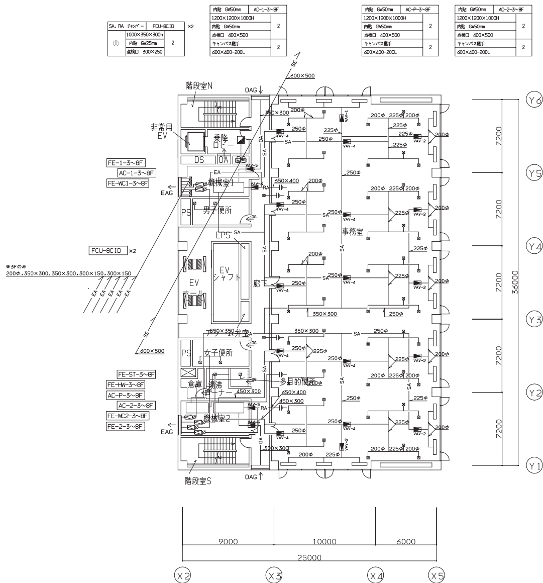
図面-空-13* 空調設備 3~8階ダクト平面図
