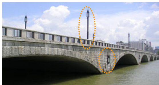
図 3-66 当時の姿に復元された萬代橋
