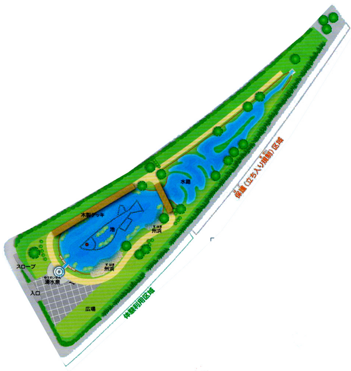
図一動物 8-1 メダカビオトップ平面図
