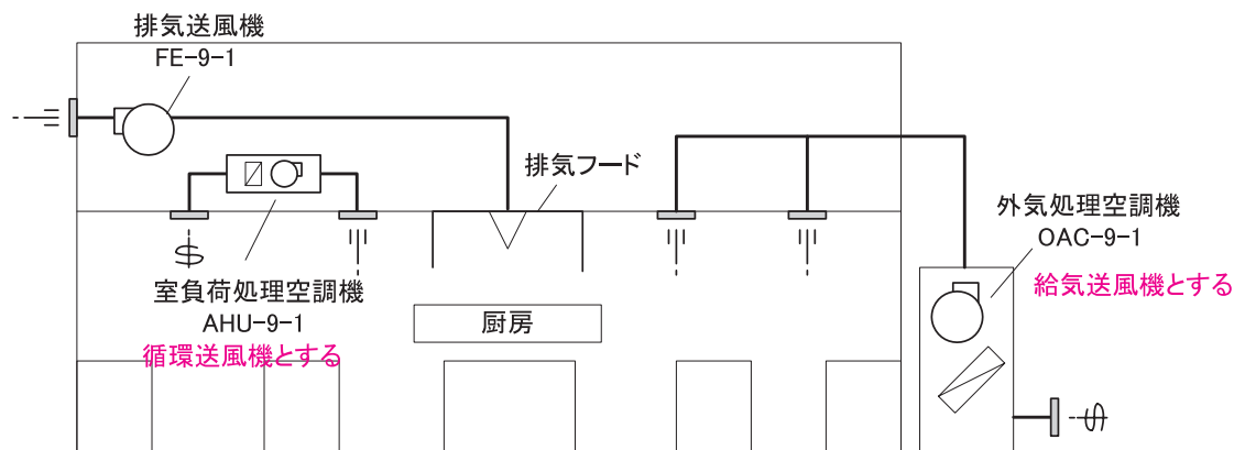
図 2-3-9 厨房空調・換気システム図
