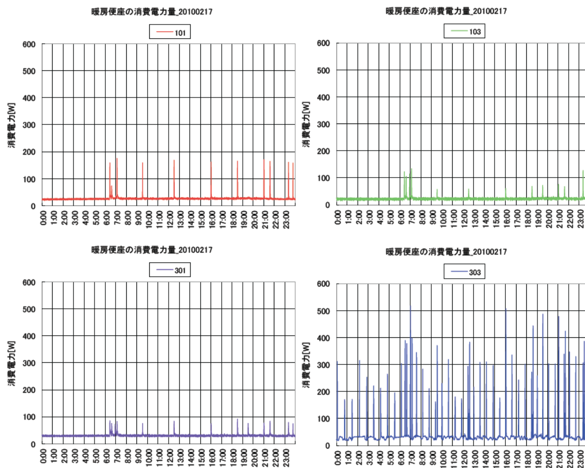
図 4.1.7 温水暖房便座の電力消費時系列データ(冬期)
