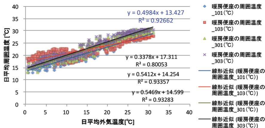
図 4.1.15 実験住宅における日平均外気温と日平均周囲温度(トイレ室温)の関係
