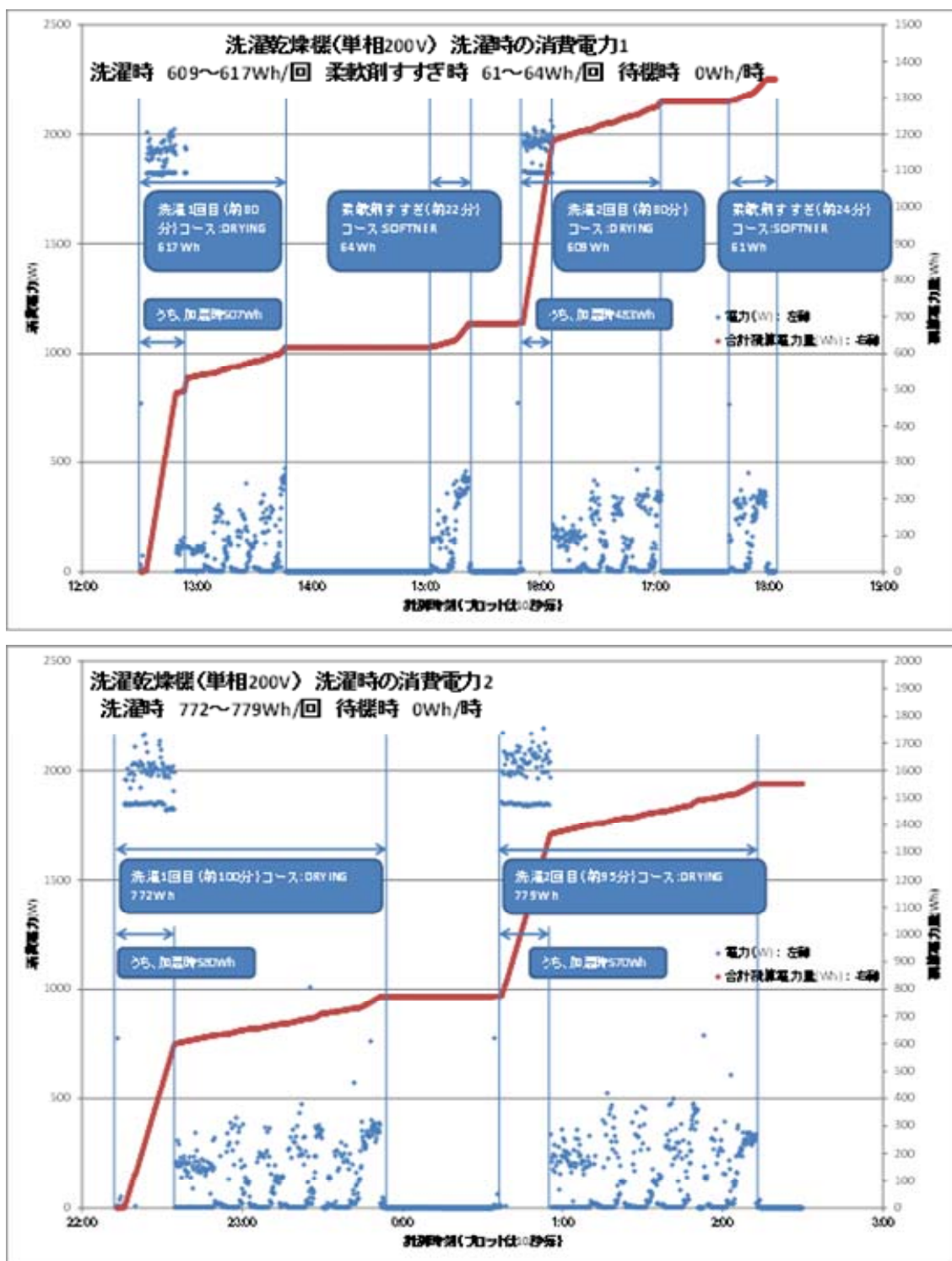
図 4.1.26 洗濯時における消費電力の変化(上図:洗濯物の少ない場合、下図:多い場合)
