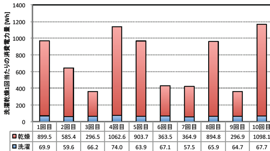
図 4.1.24 洗濯・乾燥各々の消費電力の内訳(単位:Wh)
