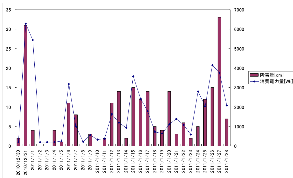
図 4.1.44 日積算積雪量と日積算消費電力
