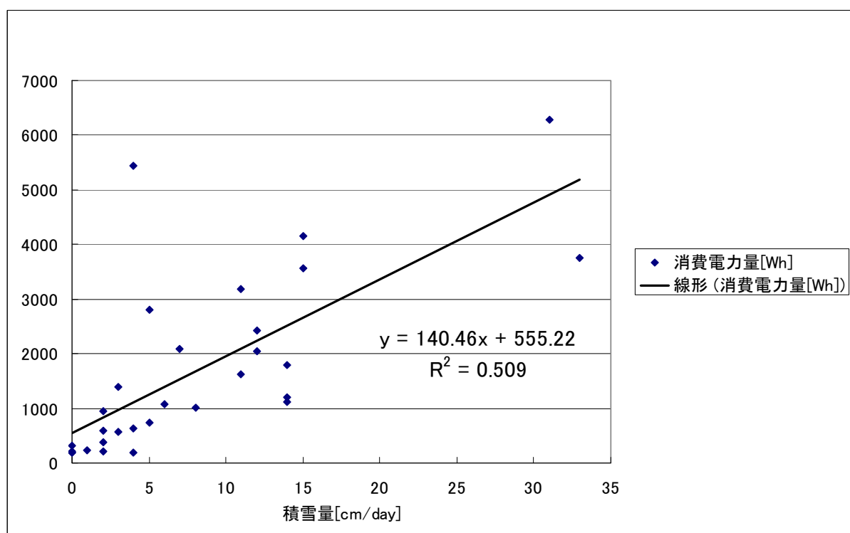
図 4.1.45 日積算積雪量と日積算消費電力の相関
