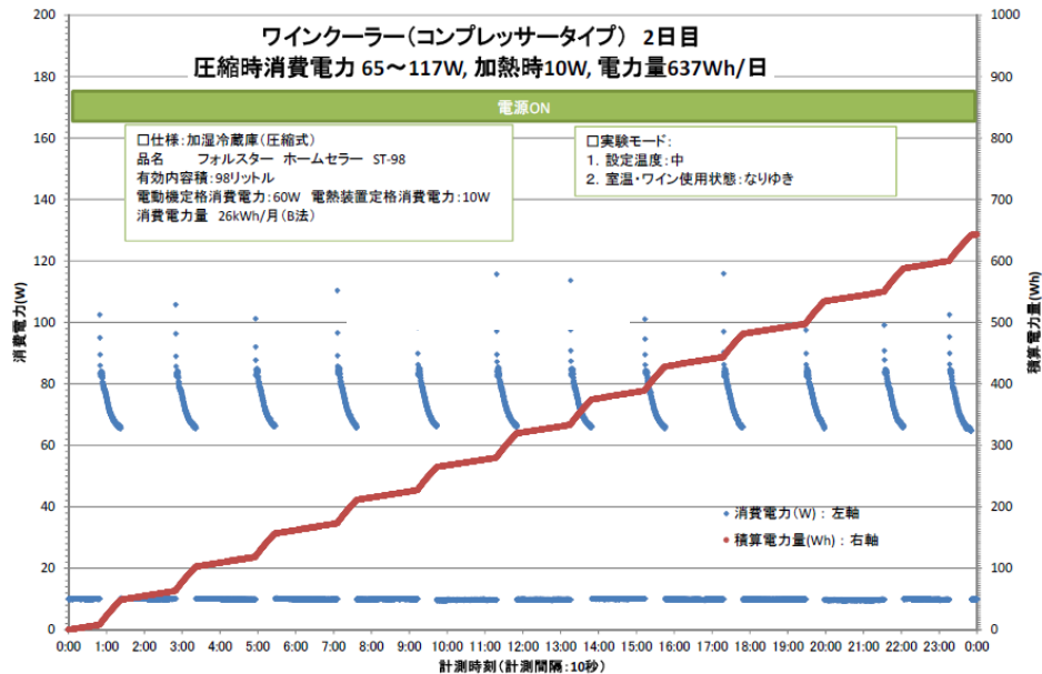
図 4.1.40 1 日の消費電力及び消費電力量の変化
