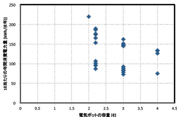
図 4.1.36 電気ポット容量と1ℓ当たりの年間消費電力量(Catalog値より換算)の関係
