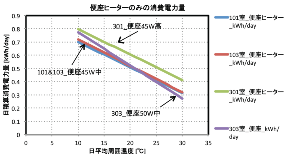
図 4.1.10 温水暖房便座の日平均周囲温度と日積算消費電力量(便座ヒーター分)の近似式 (修正前)
