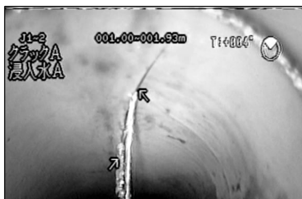
写真-1 クラックと浸入水
