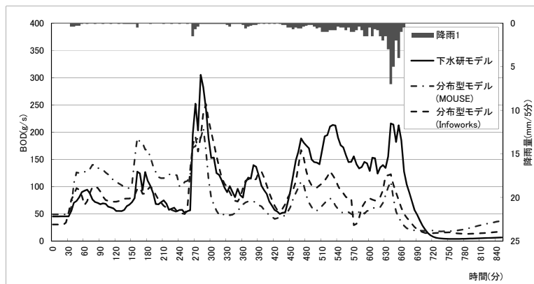
図－13 各モデルの BOD 汚濁負荷流出量解析結果の比較 (総降雨量：63mm)
