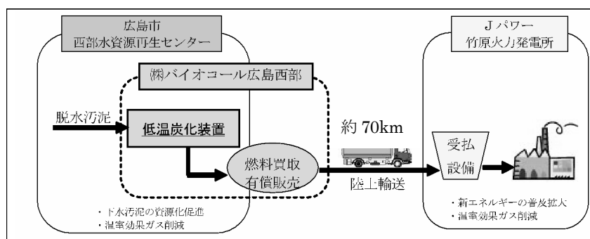
図- 10 広島市西部水資源再生センター下水汚泥燃料化事業フロー
