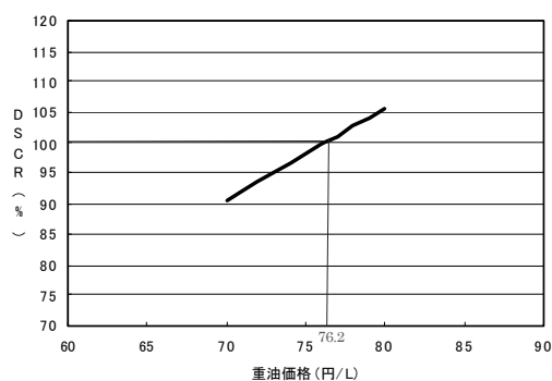
図-7 事業成立分岐点
