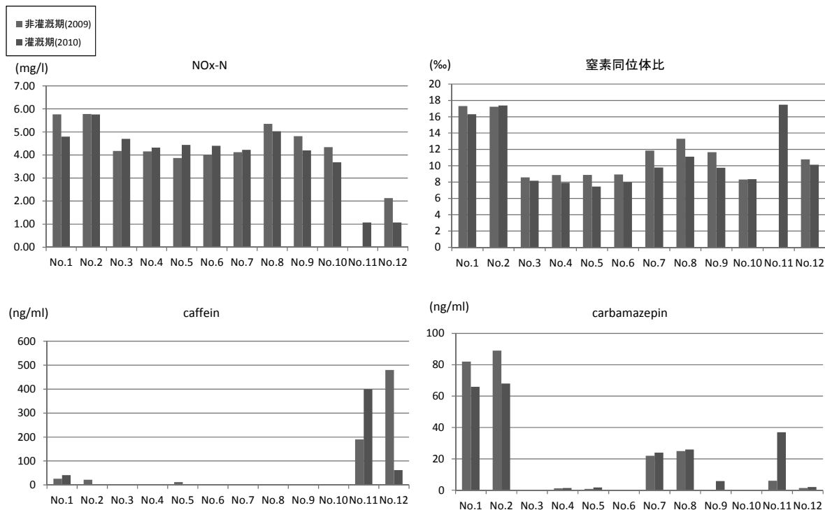
図-2 調査対象地点における水質分析結果
