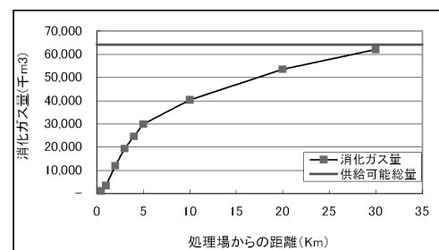
図-5 化学工業～処理場間距離と累積資源量の関係
