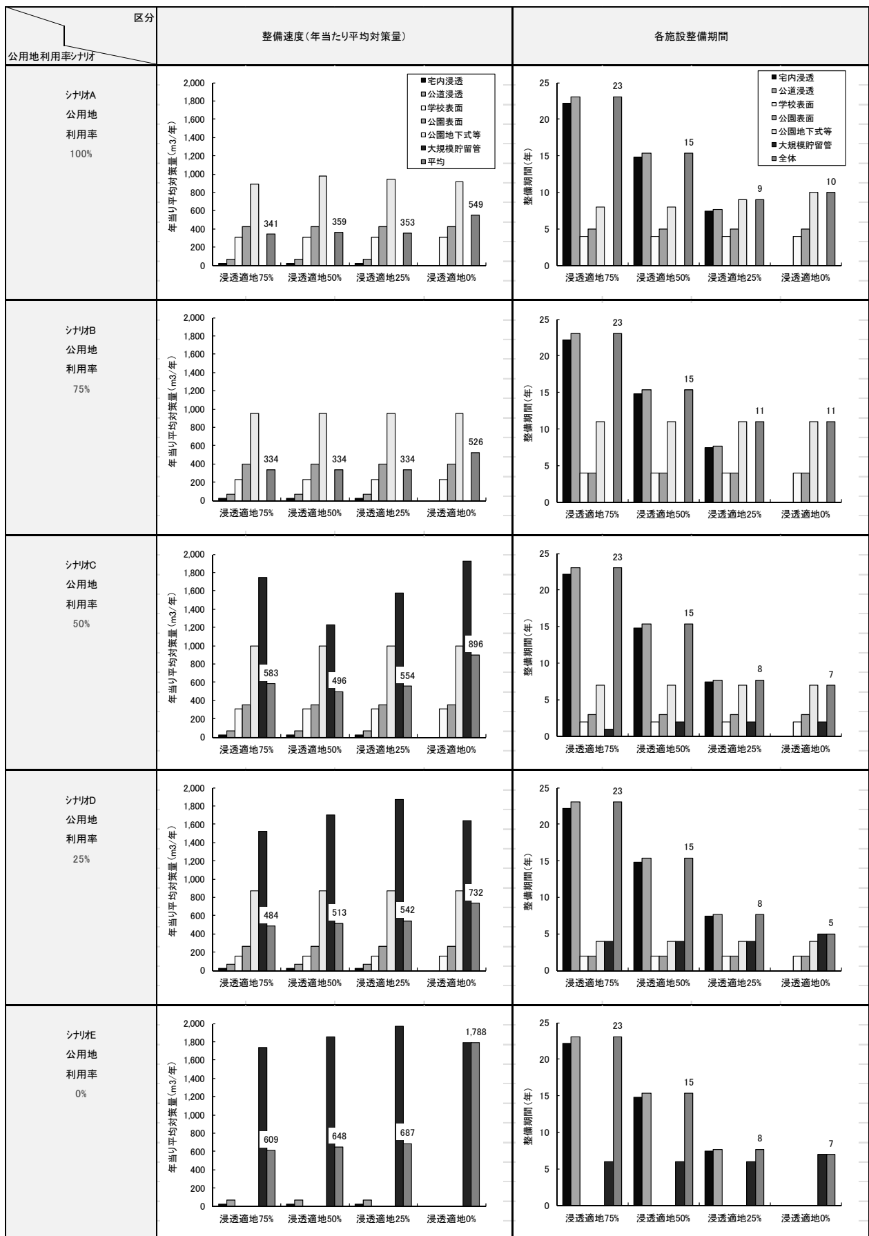
図-7 各シナリオにおける雨水貯留浸透施設の整備期間算定結果
