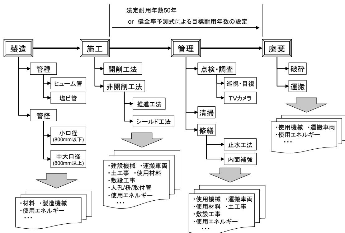
図-10 単純シナリオにおける LCA 試算対象
