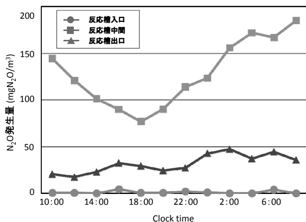
図 2 反応槽内における \text{N}_2\text{O} 発生量
