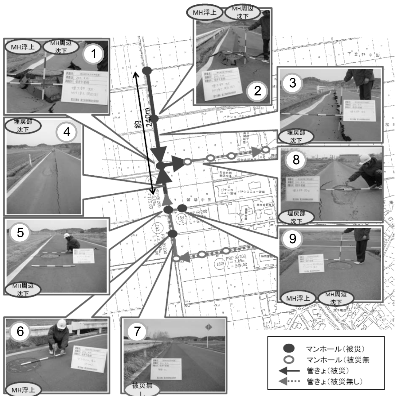
図－１ 平成 23 年東北地方太平洋沖地震による被害
