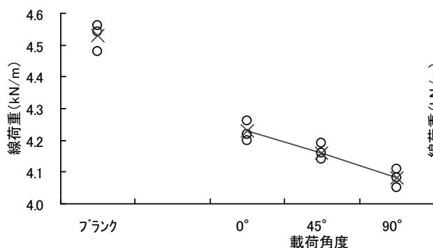
図-10 せん孔のみの試験結果
