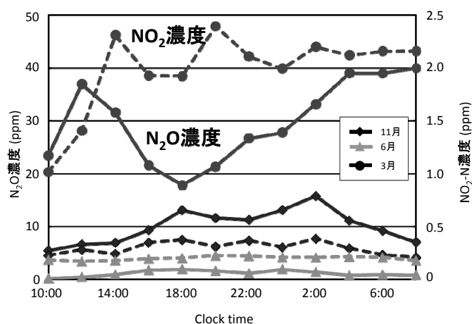
図 3 \text{N}_2\text{O} 発生量の季節変動
