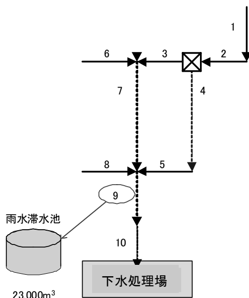
図-11 解析対象地区の概要図
