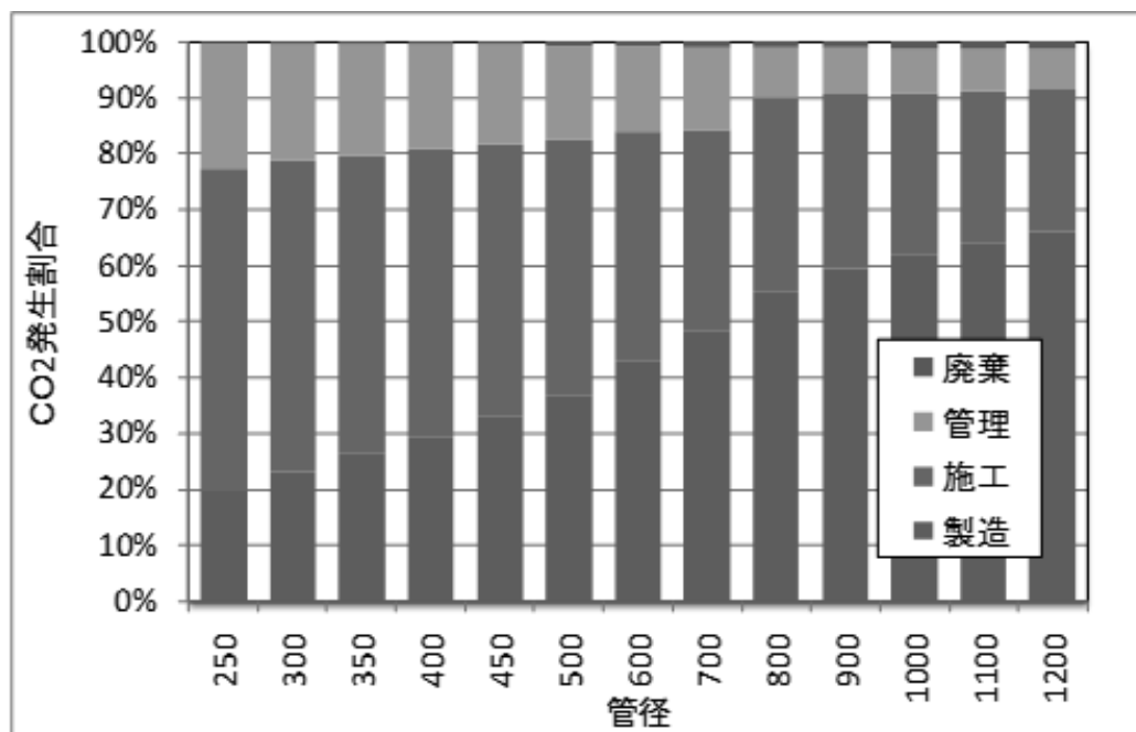
図-14 コンクリート管の工程別 CO 2 発生割合 (開削工法)
