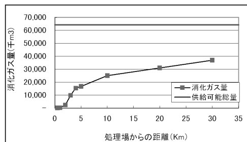
図-4 発電所～処理場間距離と累積資源量の関係
