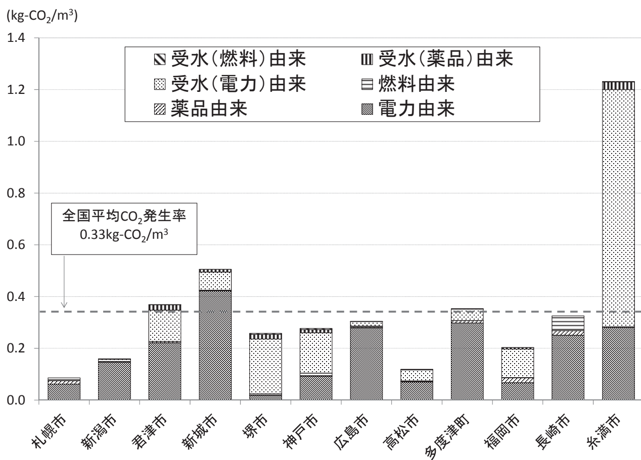
図-1 各都市におけるの水供給に係る CO 2 発生率
