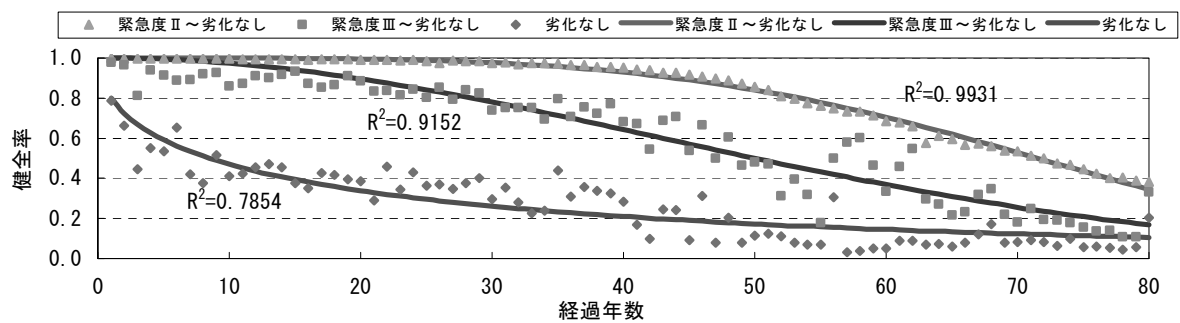
図-3 健全率曲線（公共下水道、全管種、ワイブル分布式）
