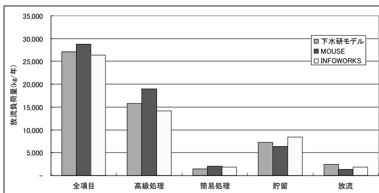
図－15 BOD 放流負荷量に関する年間解析結果の比較
