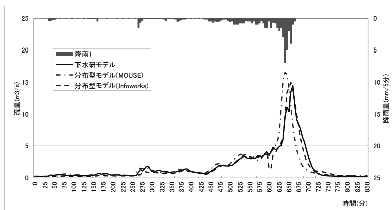
図-12 各モデルの雨水流出量解析結果の比較 (総降雨量：63mm)
