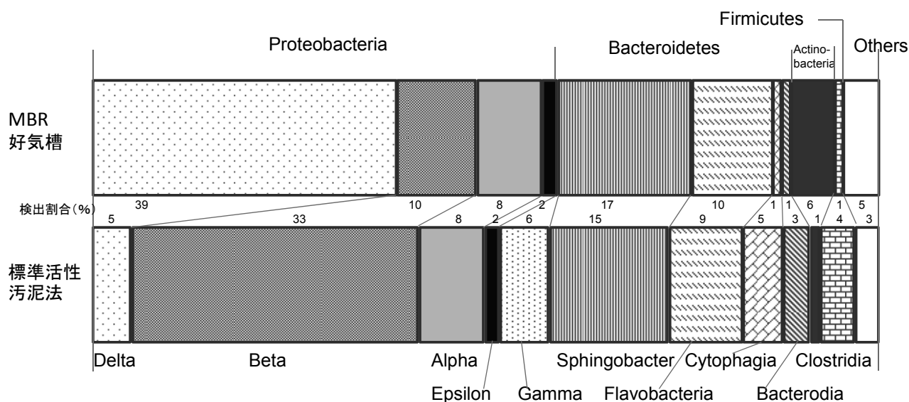
図 6 A 市下水処理場における処理法別の菌相(真正細菌)
