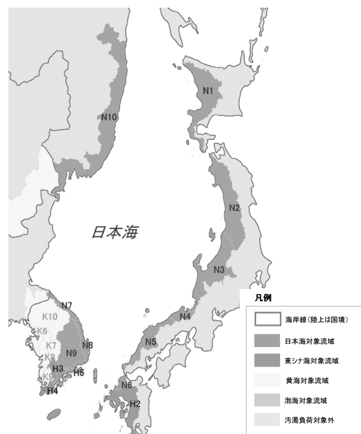
図-6 日本・韓国・ロシアにおける流域ブロック分割
