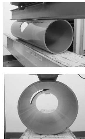
図-9 荷重の様子
