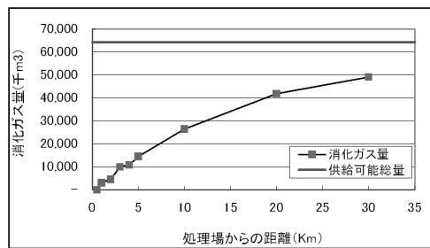
図-6 窯業・土石製品製造業～処理場間距離と累積資源量の関係
