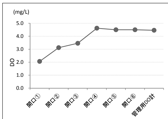
図-3 DO 測定位置と DO 濃度の分布
