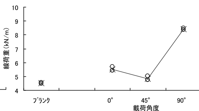
図-11 支管 1 箇所設置の試験結果
