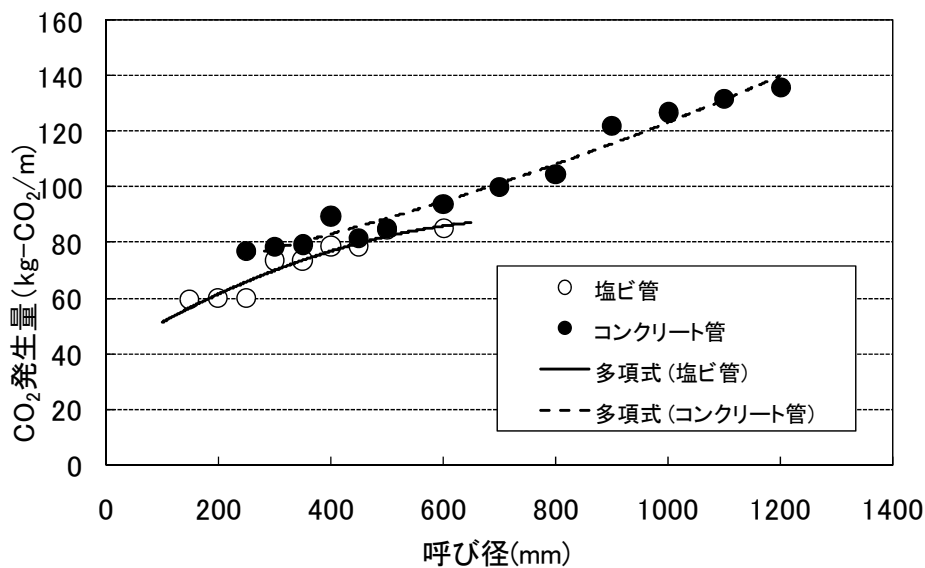
図－12 コンクリート管と塩ビ管の施工工程におけるm当たり CO 2 発生量
