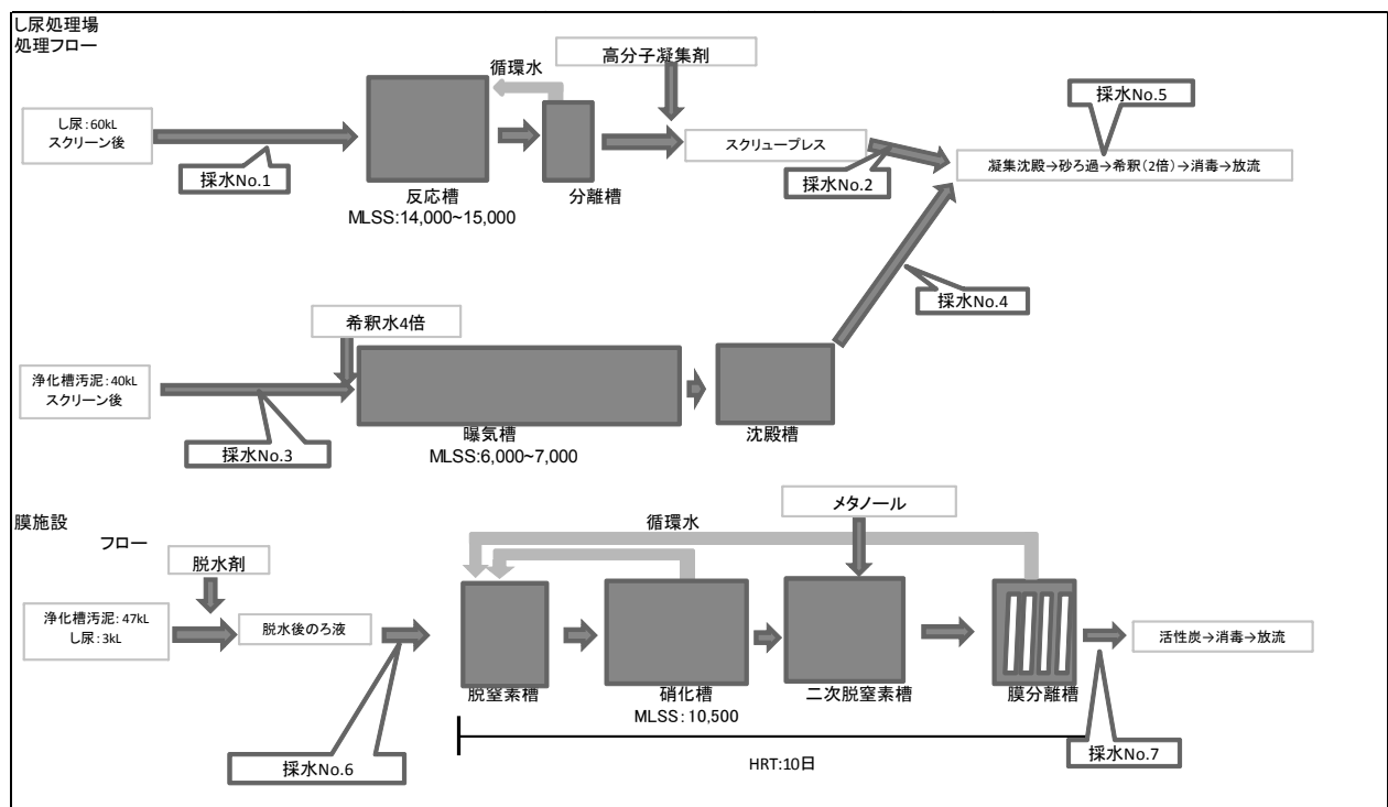
図-1 し尿処理施設における処理フローの概要及び採水地点
