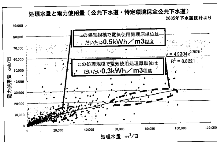
グラフ1 下水処理場の処理水量と電気使用量
