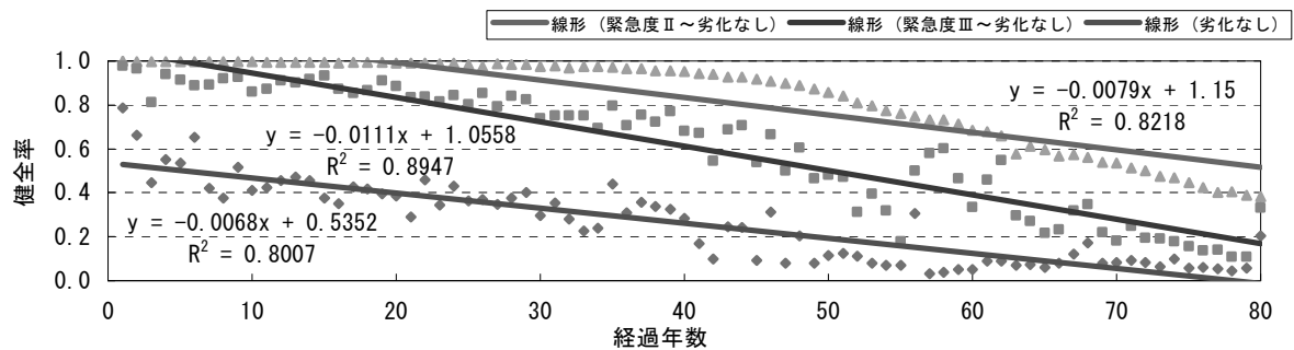
図-2 健全率曲線（公共下水道、全管種、直線式）
