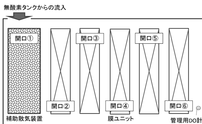
図-2 好気タンク内の DO 測定位置
