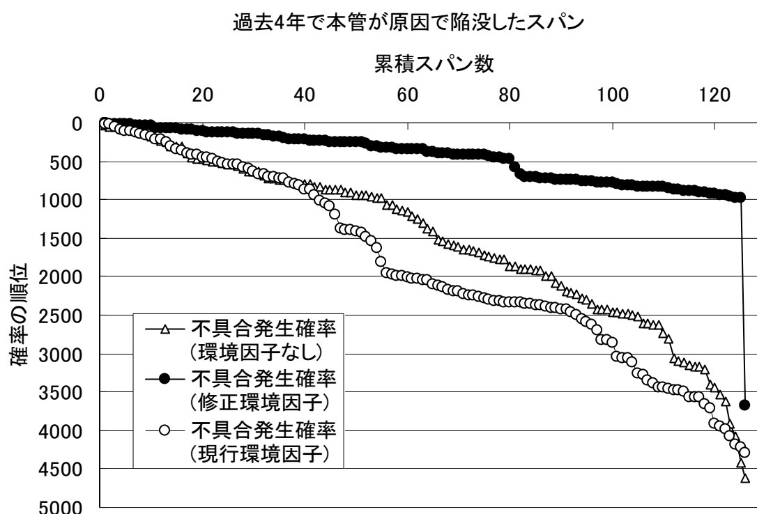
図-9 道路陥没が発生したスパンの不具合発生確率の順位と累積スパン数
