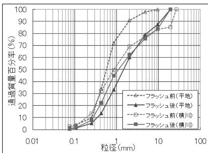
図－2 堆積物の粒径加積曲線
