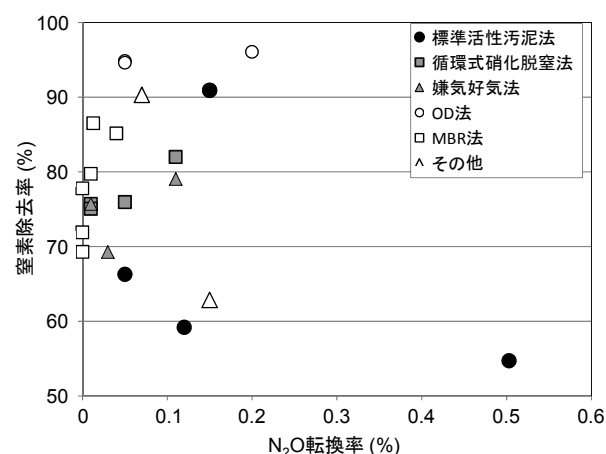
図 5 処理方式別 N_2O 転換率および窒素除去率
