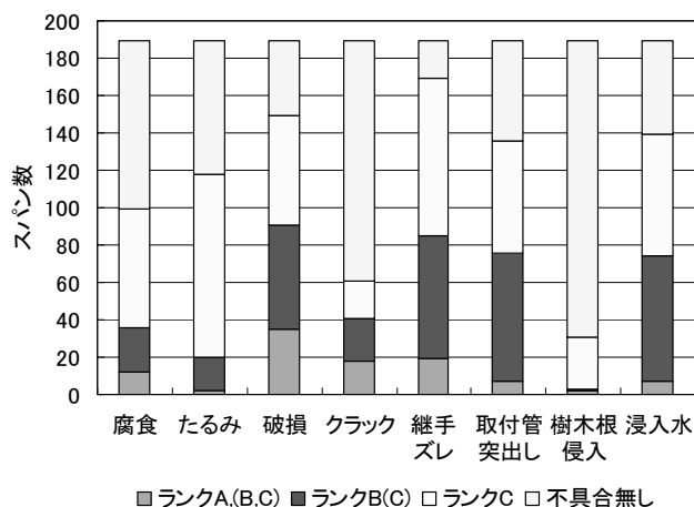
図-4 平成19年度調査における管きよの不具合
