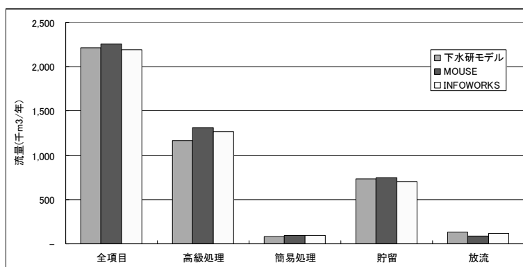
図－14 流量に関する年間解析結果の比較
