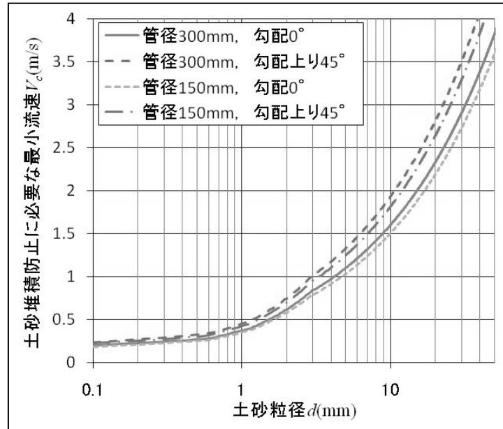
図－3 土砂掃流に必要な流速
