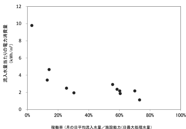
図-4 MBR の電力消費率と稼働率
