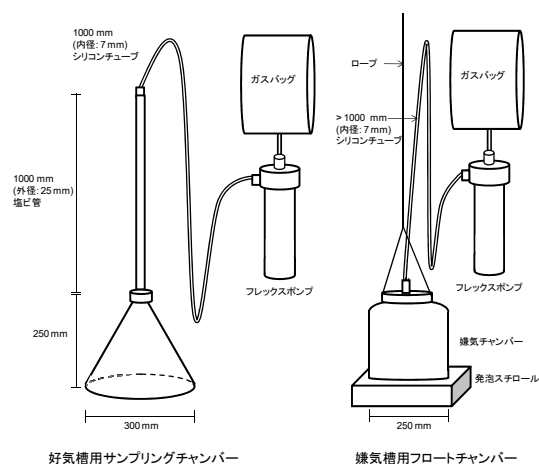
図 1 ガス捕集器
