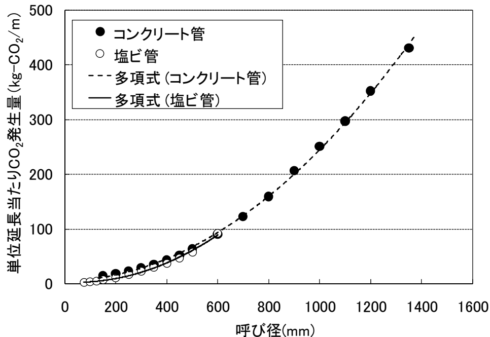
図-11 コンクリート管 (A-1) と塩ビ管 (K-1) の製造工程におけるm当たり CO 2 発生量
