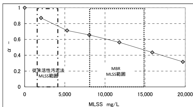
図-1 α と MLSS の関係
