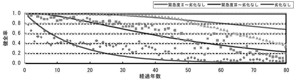
図-4 健全率曲線（公共下水道、全管種、マルコフ推移確率）
