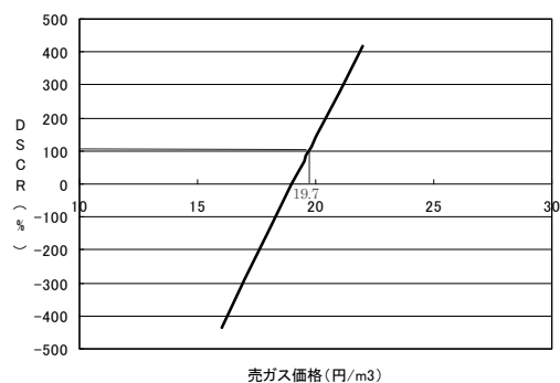
図- 8 事業成立分岐点
