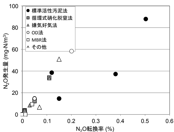
図 4 処理方式別 N_2O 転換率および N_2O 発生量
