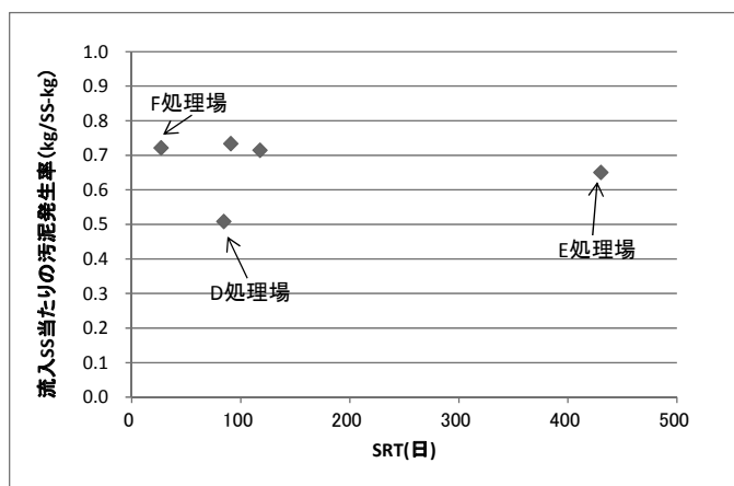
図-6 流入 SS あたりの汚泥発生率と SRT の関係
