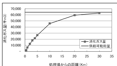
図-3 ごみ処分業～処理場間距離と累積資源量の関係
