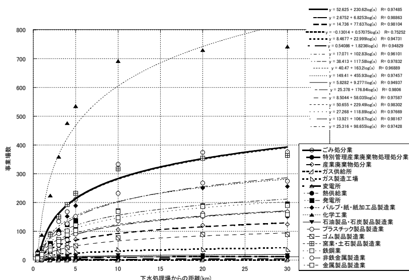
図-1 下水処理場から事業場までの距離と累計事業場数
