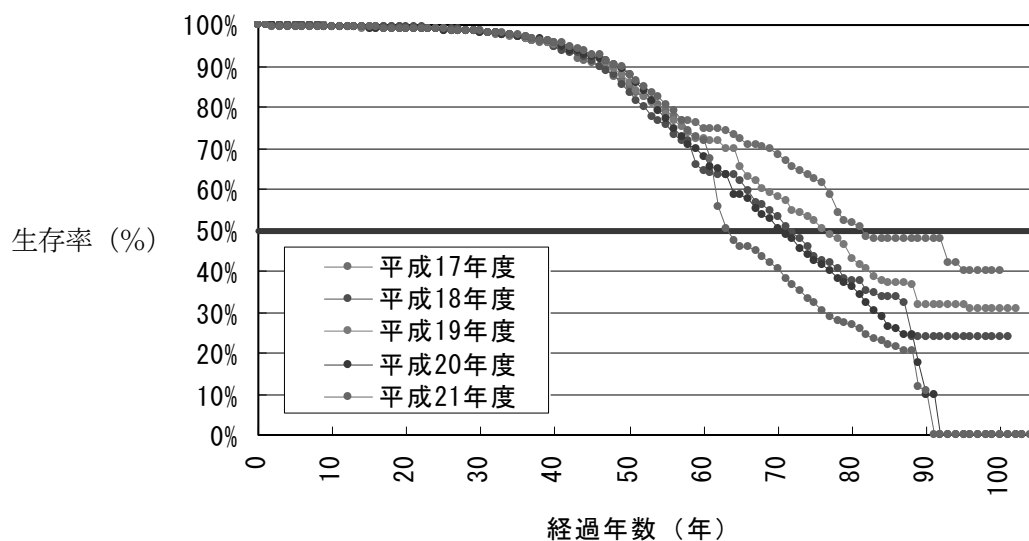
図－1 生存率（全管種：年度別）
