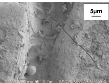
(j) VU 15 年屋外曝露(表面)
