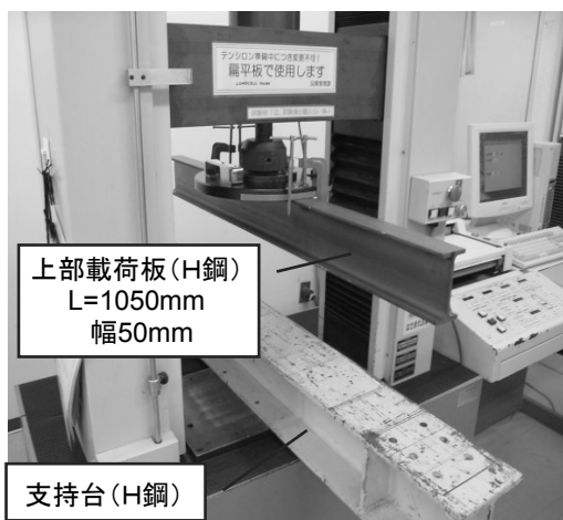
図-8 テンシロン圧縮試験機 UCT-10T
