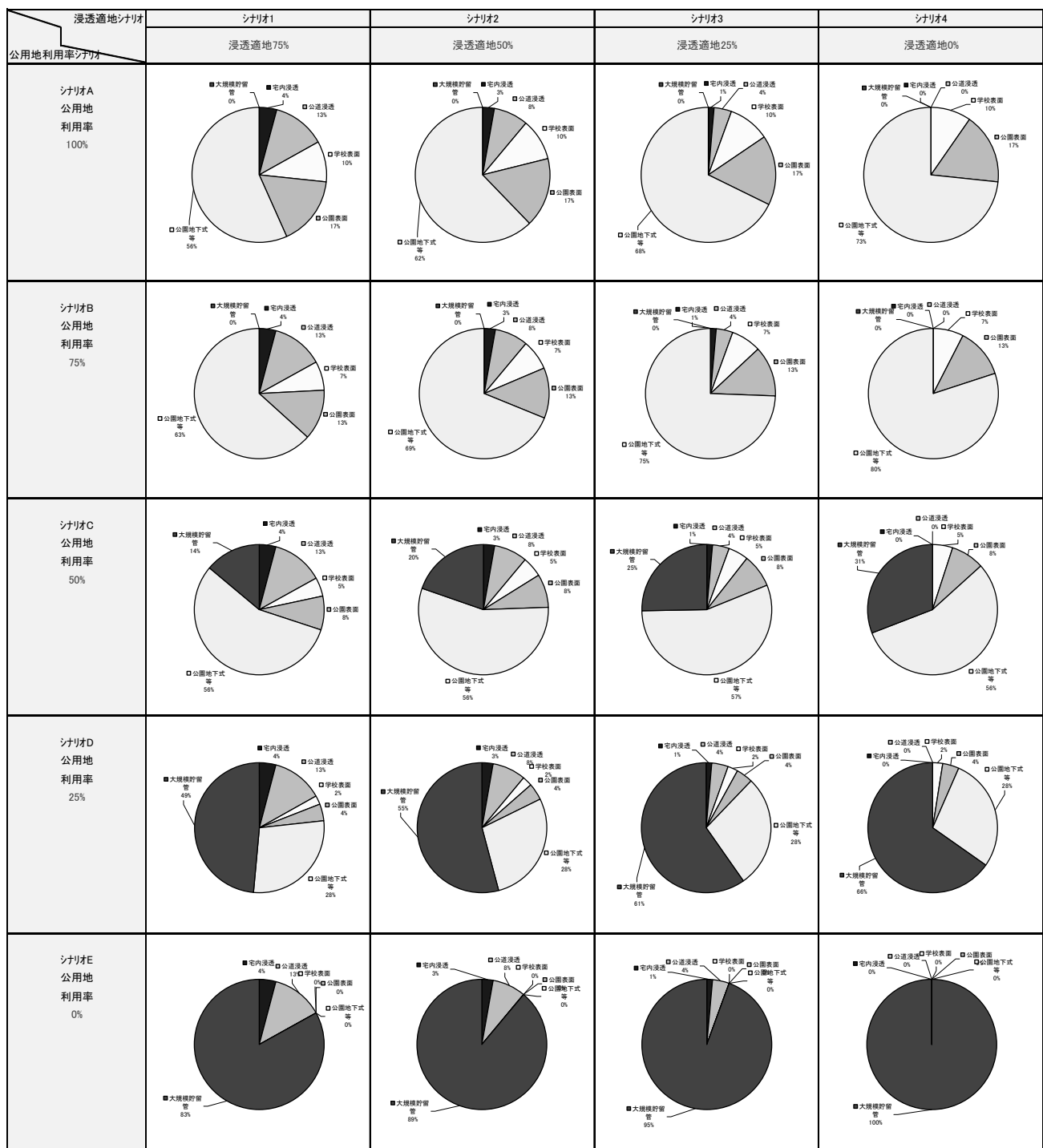
図-5 各シナリオにおける雨水流出抑制量(必要な貯留浸透量 12,519m 3 )の内訳
