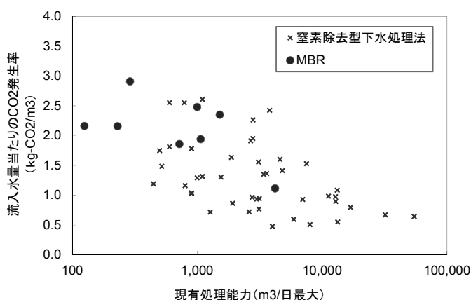
図-5 電力消費率と施設能力
