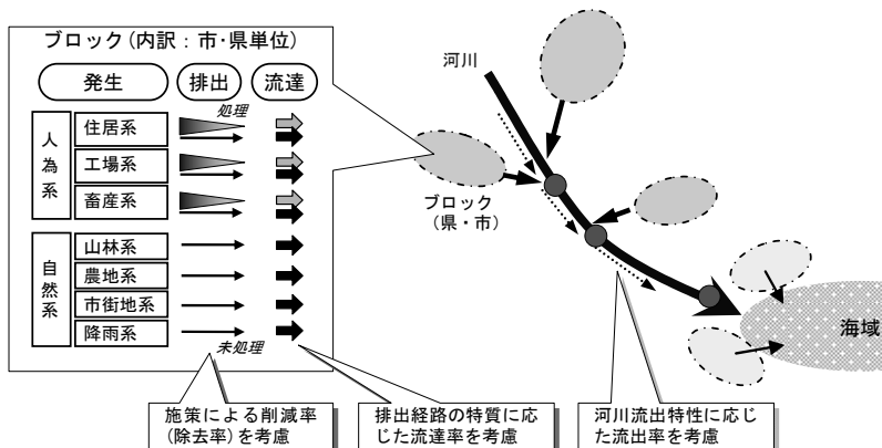
図-3 陸域からの汚濁負荷モデルの計算イメージ
