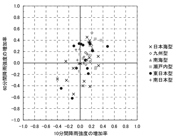
図-1 毎年 10 分最大降雨量と毎年 60 分最大降雨量の 50 年後の増加率の関係（5 年確率）
