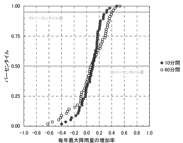
図-2 毎年 10 分最大降雨量と毎年 60 分最大降雨量の 50 年後の増加率の分布（5 年確率）
