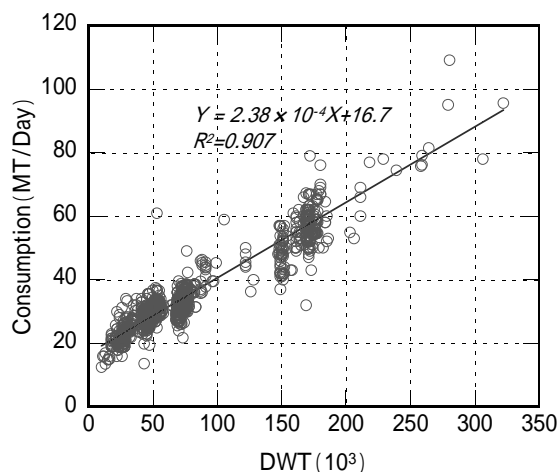
図-3.2 DWT と燃料消費量の関係 (外航船)
