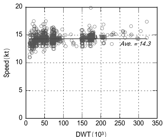
図-3.1 DWT と船速の関係 (外航船)
