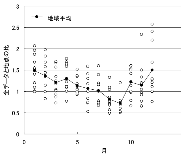
図－4.5 月降水量標準偏差の GCM20/地上アメダスにおける（全データ）と（地点）の比
