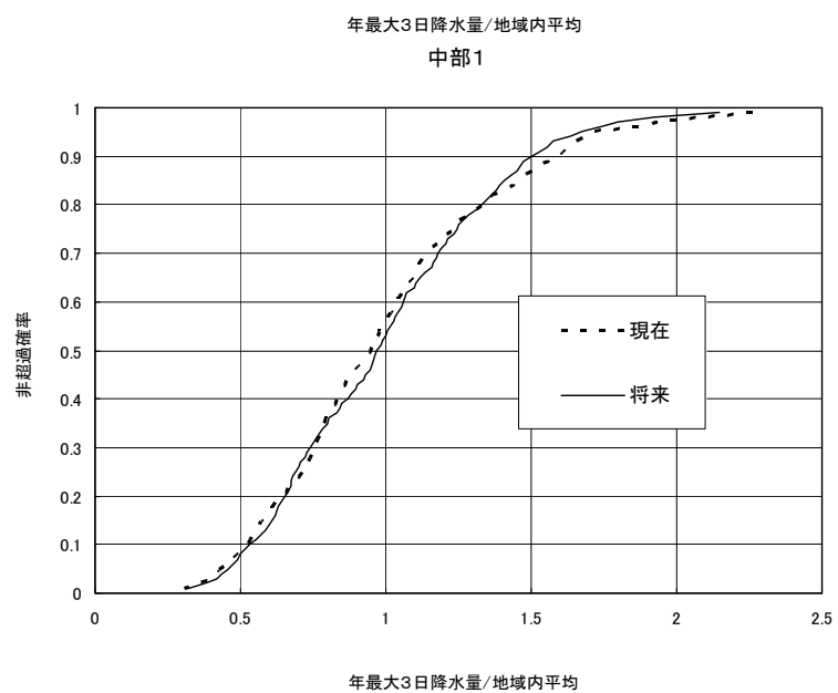
参考図－9.6 地域内平均値で無地元化した地域別確率分布（GCM20、年最大3日降雨量）
