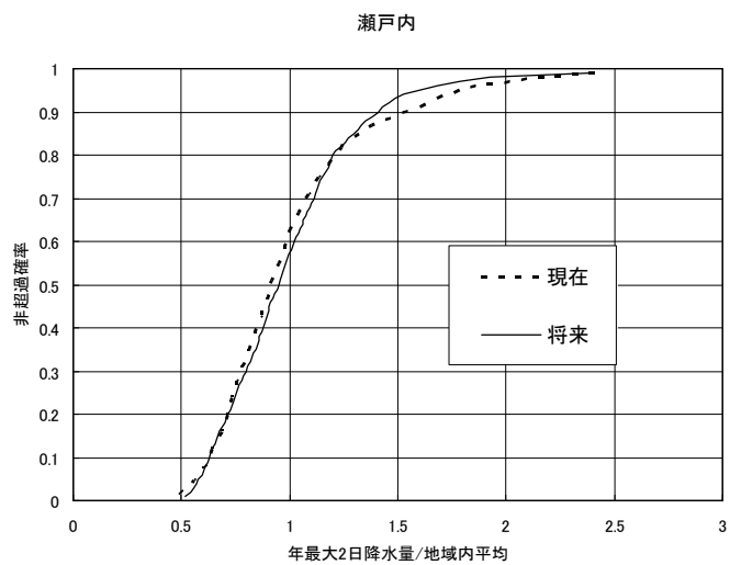
参考図－8.3 地域内平均値で無地元化した地域別確率分布（GCM20、年最大2日降雨量）
