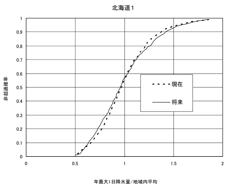
参考図－7.4 地域内平均値で無地元化した地域別確率分布（GCM20、年最大1日降雨量）
