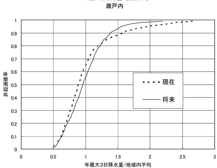
参考図－9.3 地域内平均値で無地元化した地域別確率分布（GCM20、年最大3日降雨量）
