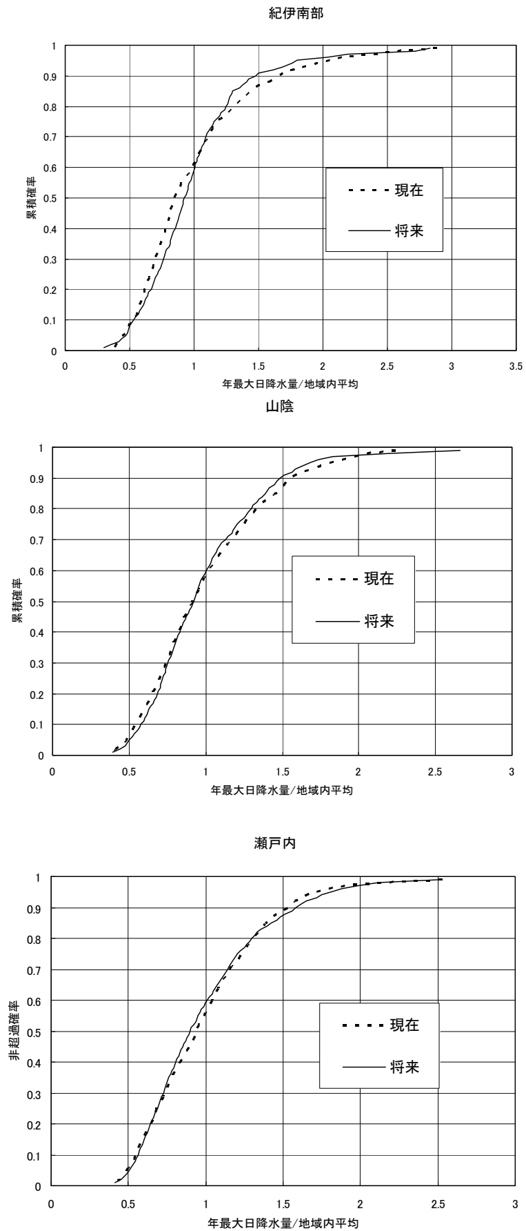
参考図－11.3 地域内平均値で無地元化した地域別確率分布（RCM20、年最大1日降雨量）
