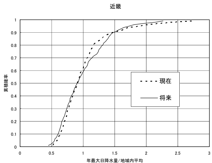
参考図－7.2 地域内平均値で無地元化した地域別確率分布（GCM20、年最大1日降雨量）
