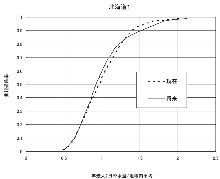
参考図－8.4 地域内平均値で無地元化した地域別確率分布（GCM20、年最大2日降雨量）
