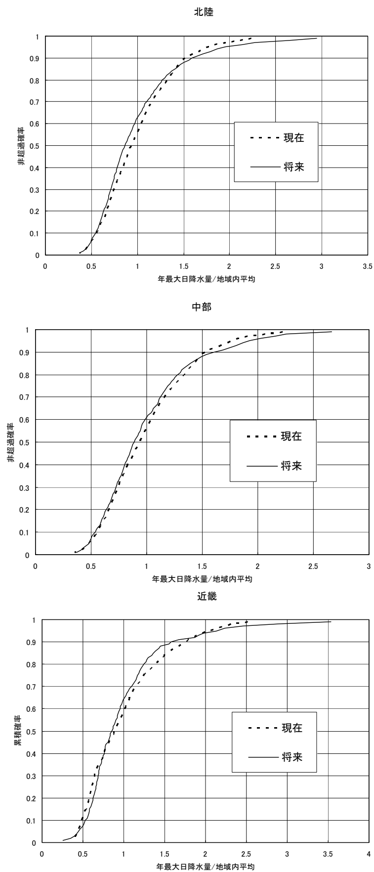
参考図－11.2 地域内平均値で無地元化した地域別確率分布（RCM20、年最大1日降雨量）
