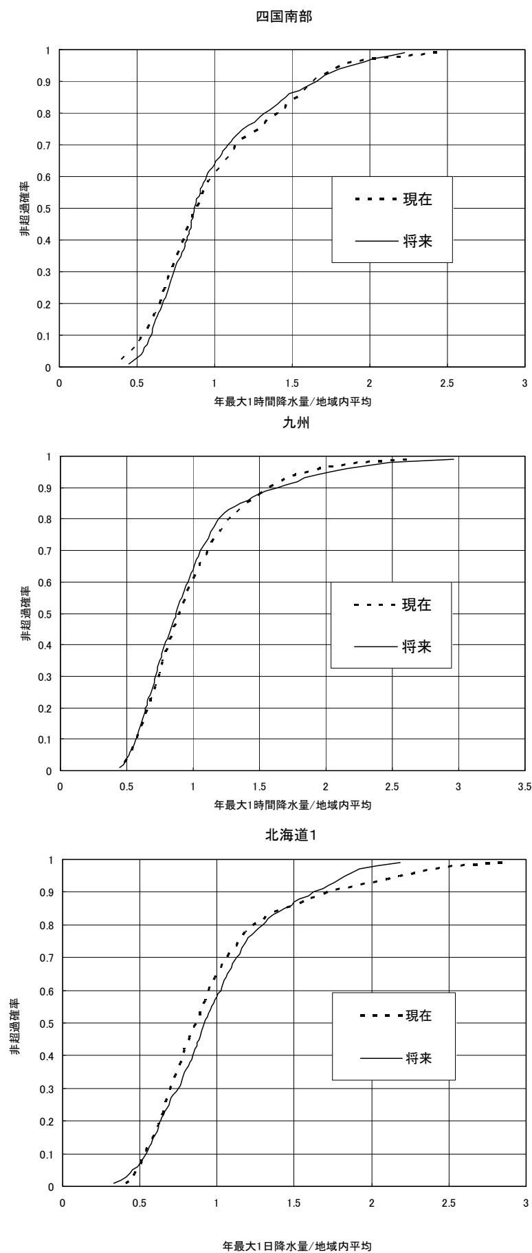
参考図－10.4 地域内平均値で無地元化した地域別確率分布（GCM20、年最大1時間降雨量）
