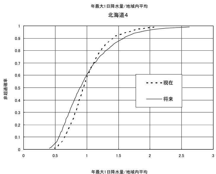
参考図－7.5 地域内平均値で無地元化した地域別確率分布（GCM20、年最大1日降雨量）
