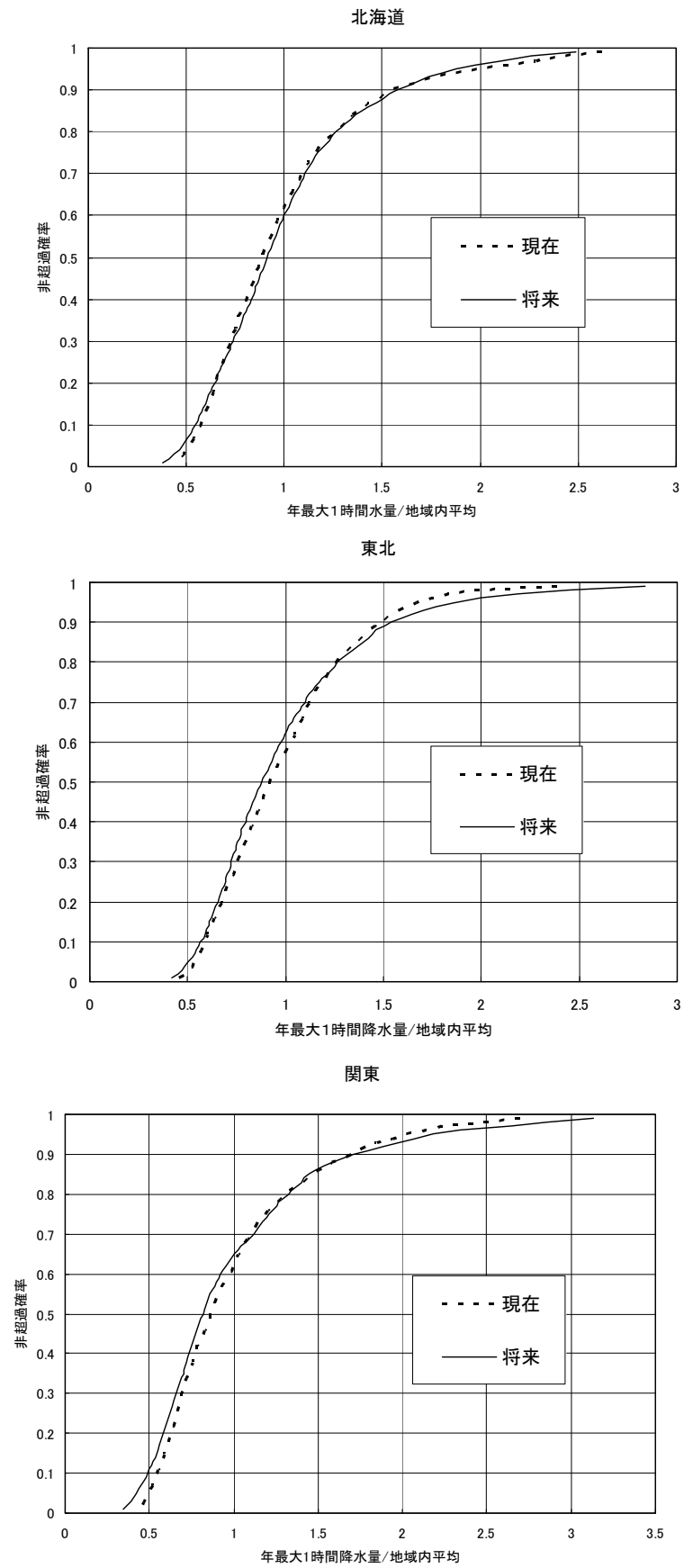
参考図－10.1 地域内平均値で無地元化した地域別確率分布（GCM20、年最大1時間降雨量）
