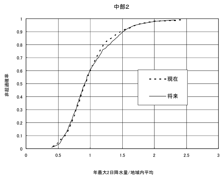
参考図－8.7 地域内平均値で無地元化した地域別確率分布（GCM20、年最大2日降雨量）
