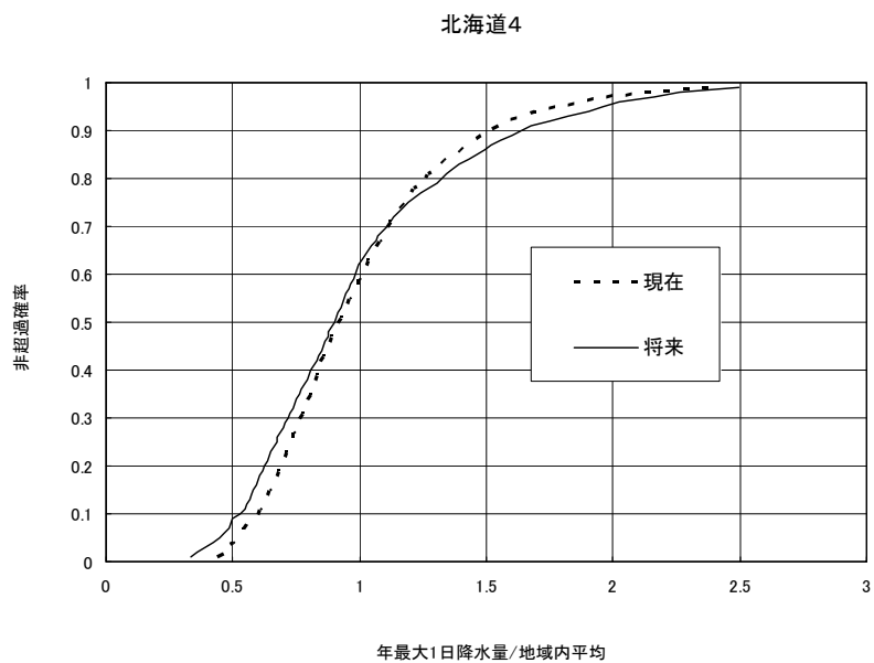
参考図－11.5 地域内平均値で無地元化した地域別確率分布（RCM20、年最大1日降雨量）
