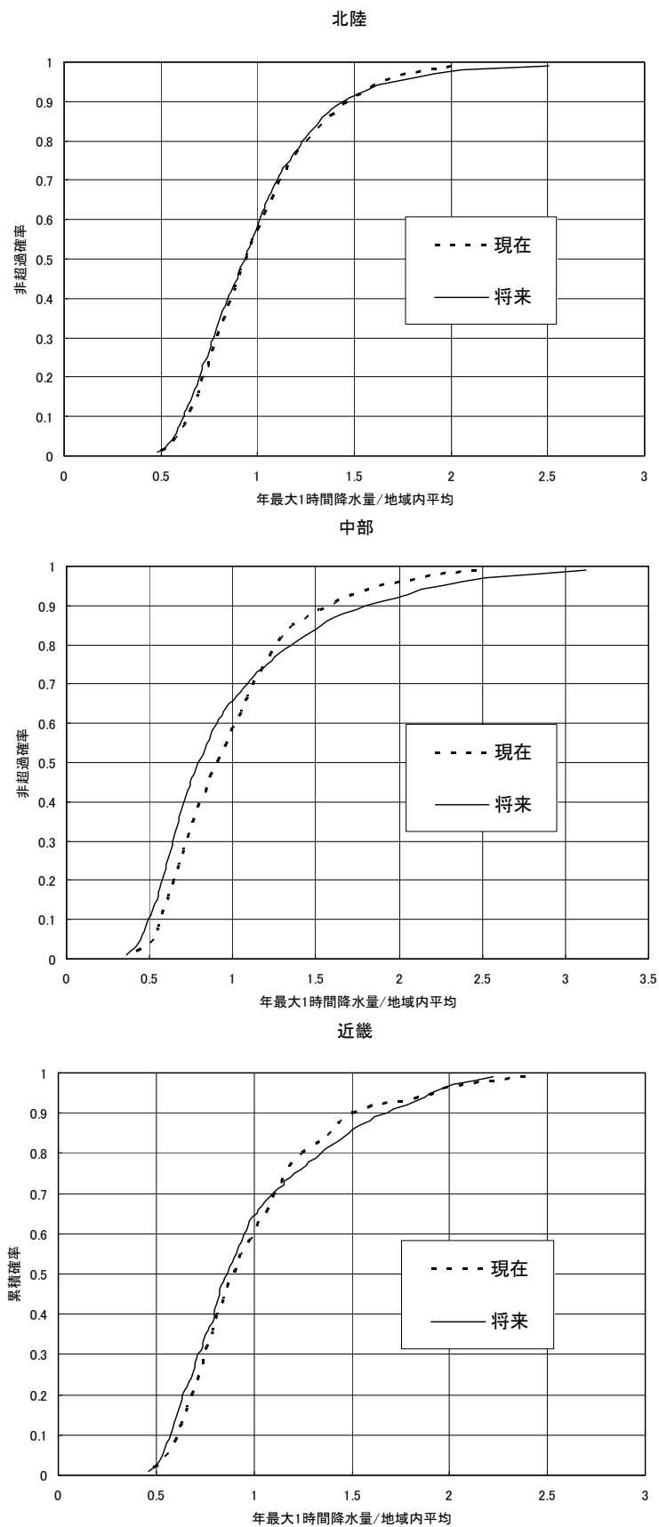
参考図－10.2 地域内平均値で無地元化した地域別確率分布（GCM20、年最大1時間降雨量）
