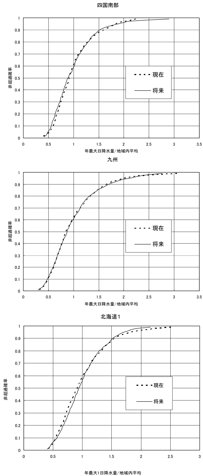
参考図－11.4 地域内平均値で無地元化した地域別確率分布（RCM20、年最大1日降雨量）
