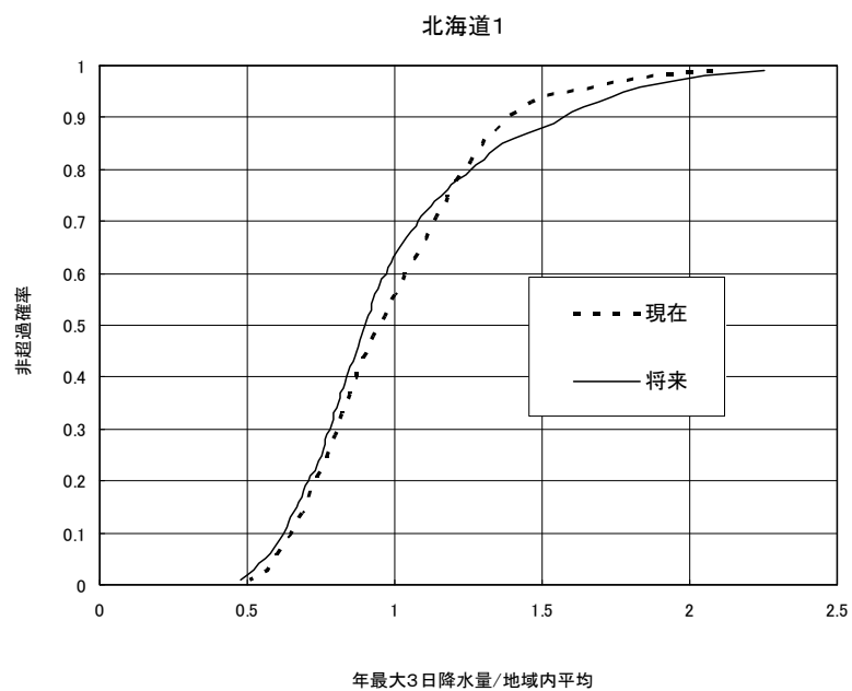
参考図－9.4 地域内平均値で無地元化した地域別確率分布（GCM20、年最大3日降雨量）
