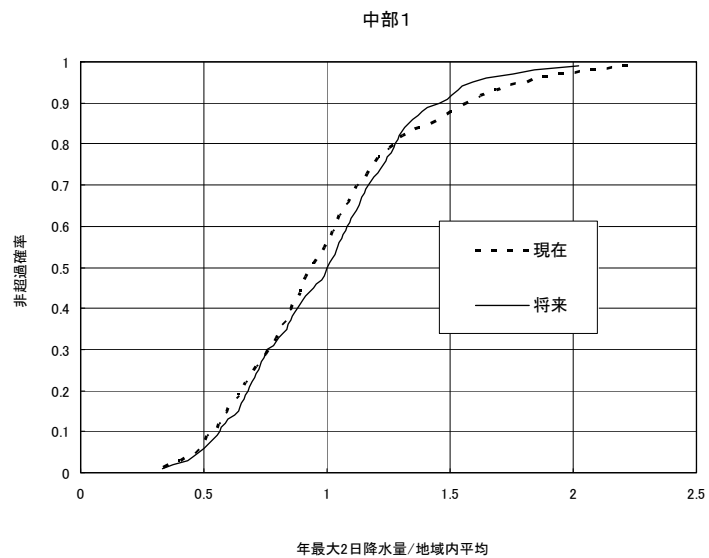
参考図－8.6 地域内平均値で無地元化した地域別確率分布（GCM20、年最大2日降雨量）
