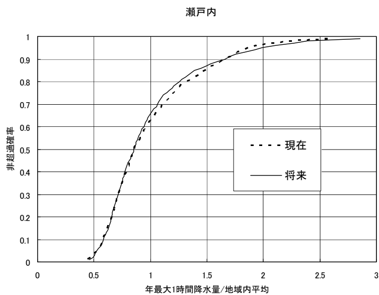
参考図－10.3 地域内平均値で無地元化した地域別確率分布（GCM20、年最大1時間降雨量）
