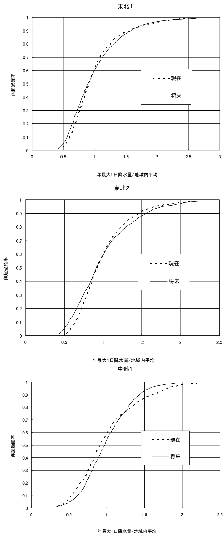
参考図－7.6 地域内平均値で無地元化した地域別確率分布（GCM20、年最大1日降雨量）
