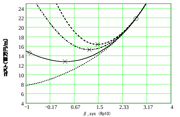
図-E.7 施工時 LCC 曲線 ( n=5 , \times : LCC 最小, \circ : 施工時標準照査, \diamond : 完成時標準照査)
