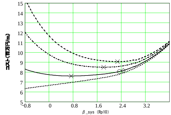
図-E.4 施工時 LCC 曲線 ( n=5 , × : LCC 最小, ○ : 施工時標準照査, ◇ : 完成時標準照査)
