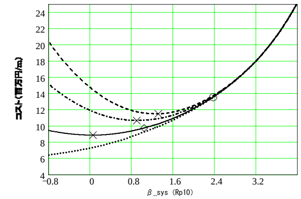
図-E.2 施工時 LCC 曲線 ( n=5 , × : LCC 最小, ○ : 施工時標準照査, ◇ : 完成時標準照査)
