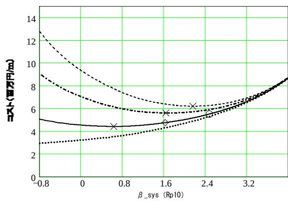
図-E.10 施工時 LCC 曲線 ( n=10 , \times : LCC 最小, \circ : 施工時標準照査, \diamond : 完成時標準照査)
