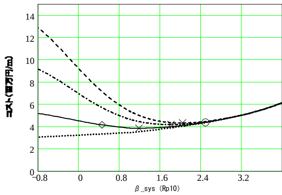
図-E.6 施工時 LCC 曲線 ( n=5 , × : LCC 最小, ○ : 施工時標準照査, ◇ : 完成時標準照査)
