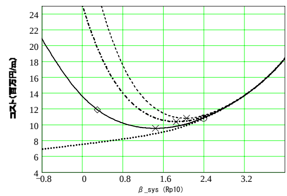
図-E.10 施工時 LCC 曲線 ( n=10 , \times : LCC 最小, \circ : 施工時標準照査, \diamond : 完成時標準照査)
