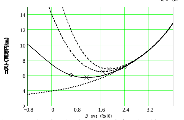
図-E.7 施工時 LCC 曲線 ( n=5 , \times : LCC 最小, \circ : 施工時標準照査, \diamond : 完成時標準照査)
