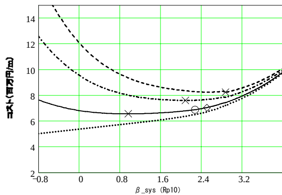
図-E.4 施工時 LCC 曲線 ( n=5 , × : LCC 最小, ○ : 施工時標準照査, ◇ : 完成時標準照査)
