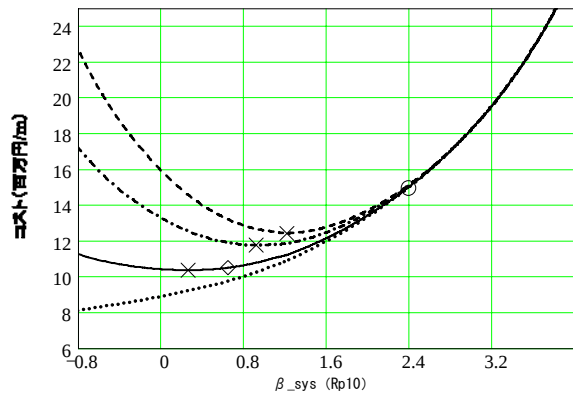
図-E.2 施工時 LCC 曲線 ( n=5 , × : LCC 最小, ○ : 施工時標準照査, ◇ : 完成時標準照査)
