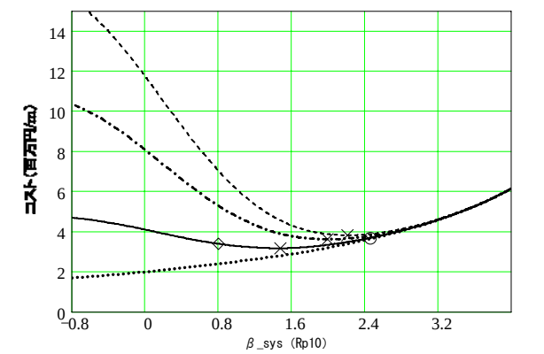
図-E.15 施工時LCC曲線 ( n=10 , \times : LCC最小, \circ : 施工時標準照査, \diamond : 完成時標準照査)
