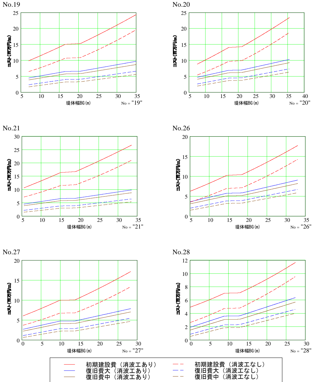
図-D.2 初期建設費と復旧費
