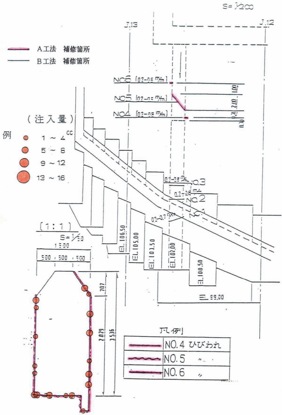
図 3.4 監査廊注入実績
