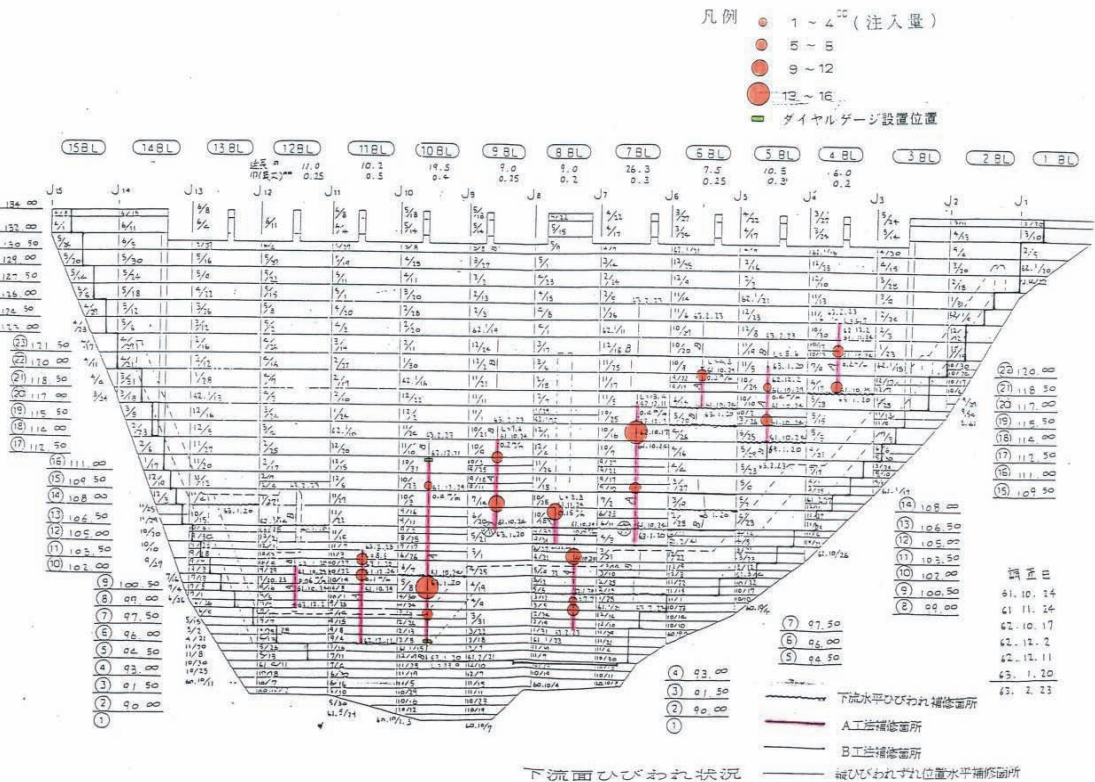
図 3.3 堤体下流面注入実績
