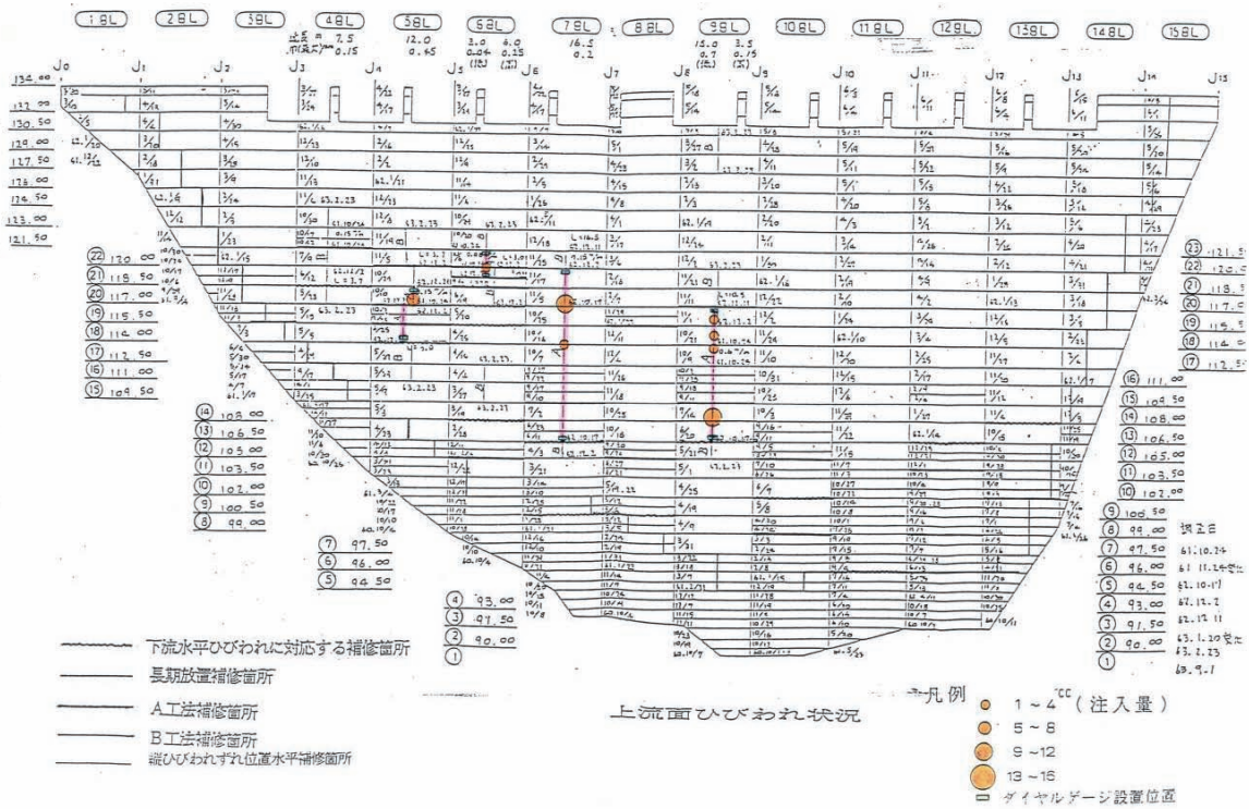
図 3.2 堤体上流面注入実績
