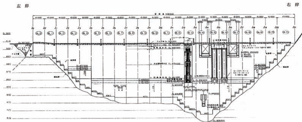
図 1.4 上流面図
