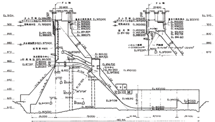
図 1.3 断面図
