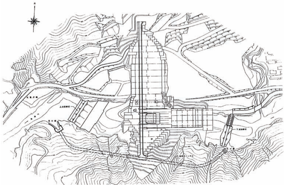
図 1.2 平面図
