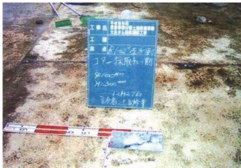
コア一抜き調査。採取コア(R1+2.0m)。
