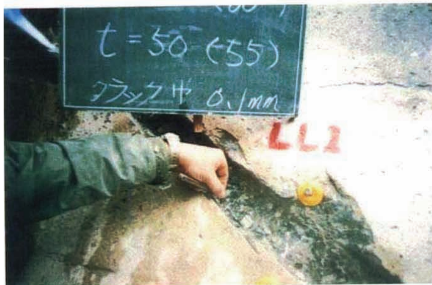
ハツリ後クラック調査(LL1+0m)。開口幅0.1mm。
