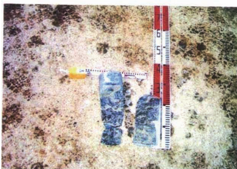
コア一抜き調査。同上フェノールフタレイン塗布前。
