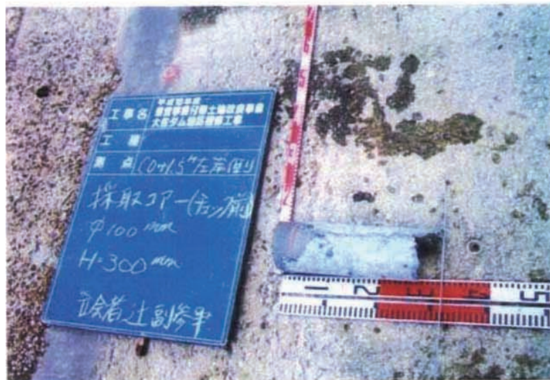
コアー抜き調査。採取コア(CL0+1.5m)。
