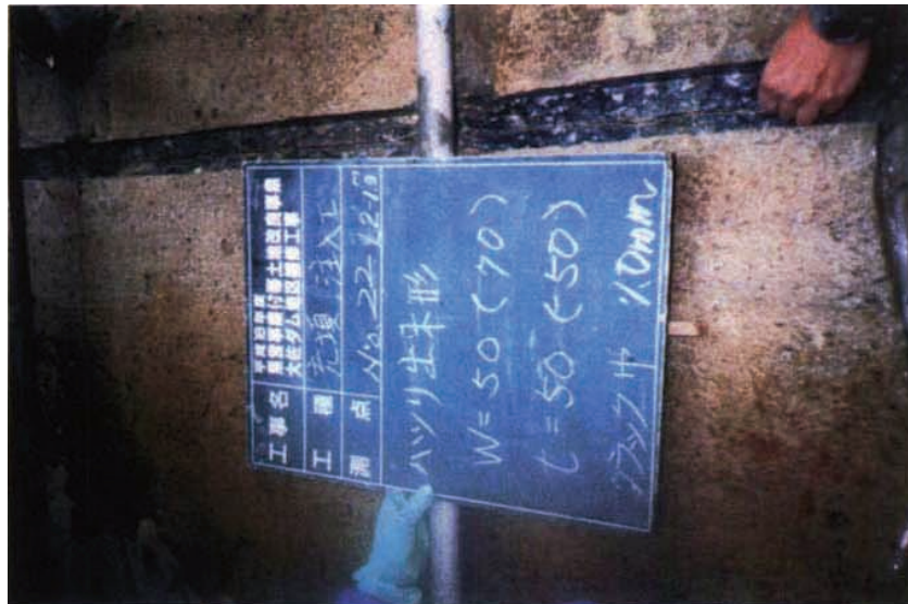
ハツリ後クラック調査(L2-1m 右岸側横断目地)。開口幅1.0mm
