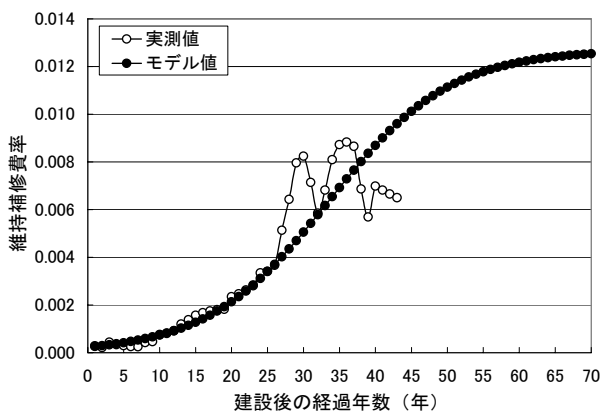
図-8(1) 維持補修費率モデル1
