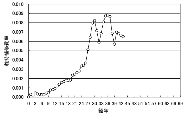
図-6(1) 維持補修費率関数 (右上り傾向有り)
