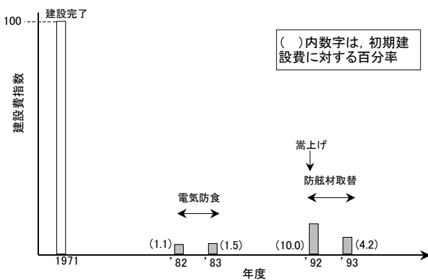
図-1 維持補修の実施例
