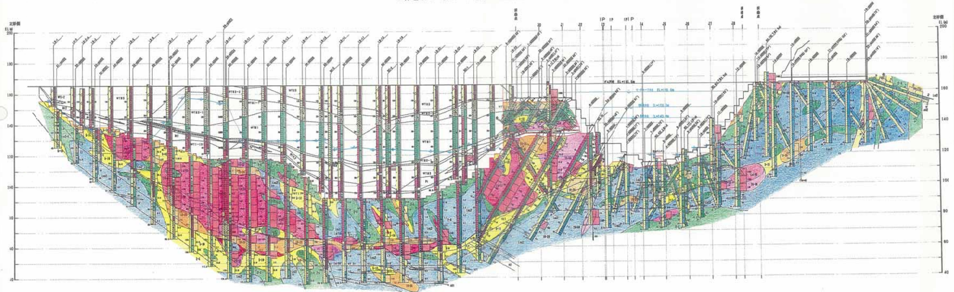
左岸直水工-主カーテン沿い ルジオンマップ
