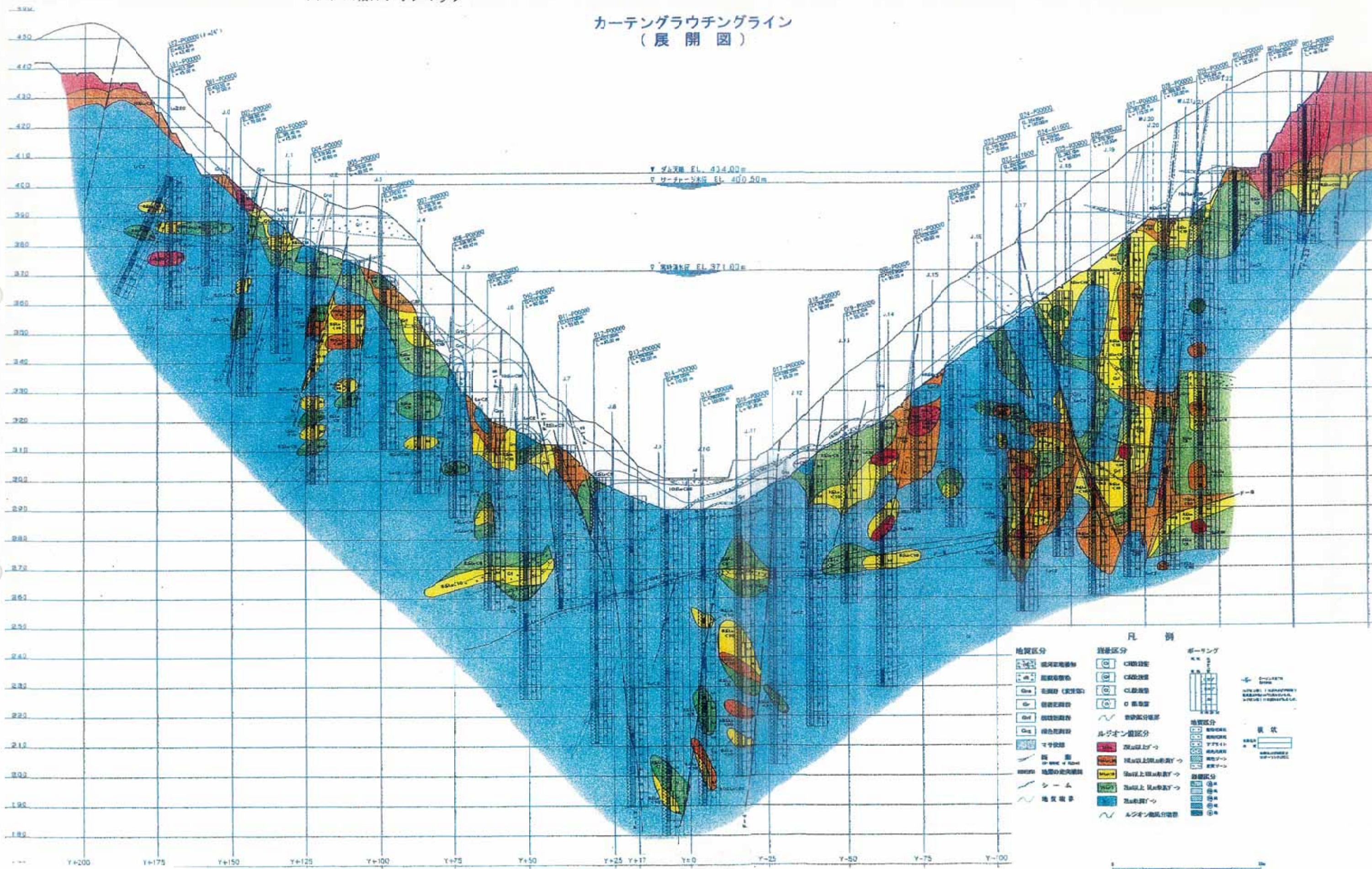
(5) ダム軸ルジオンマップ
