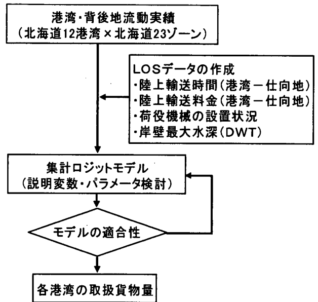
図-41 港湾選択モデルの構築フロー
