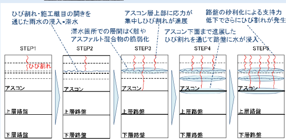
アスファルト舗装の早期劣化メカニズムの一例
