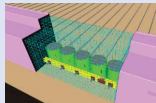
< CIMモデル(栈橋) >
