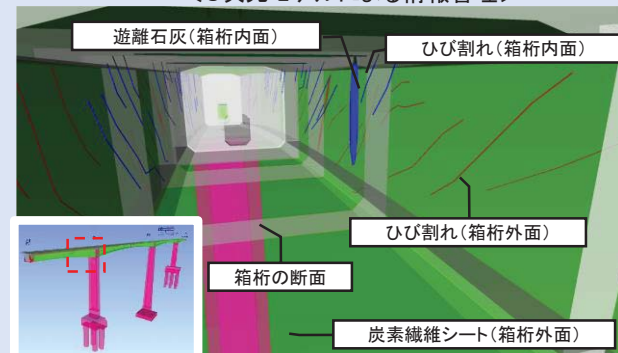
< 3次元モデルによる情報管理 >
