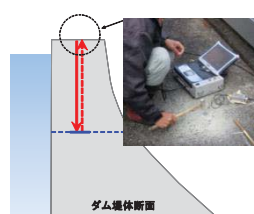
反射波・伝搬速度を計測しひび割れ等の変状を特定
