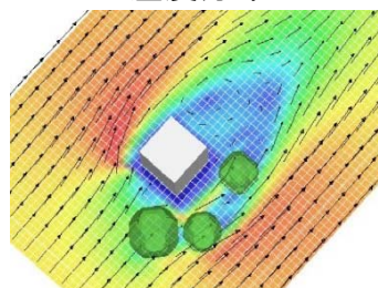
風と熱の流れの解析
