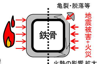
地震被害(亀裂)の影響
