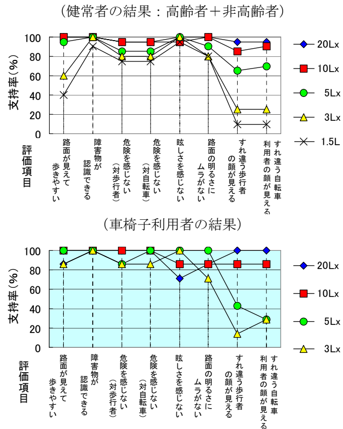
図5-4 歩行者用照明の照明レベルごとの視認性評価結果
