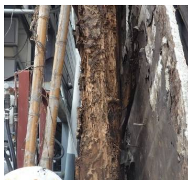
写真 46 写真 45 の柱の生物劣化
