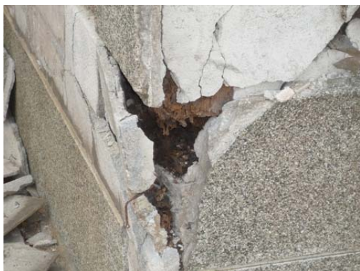
写真9 写真8柱脚部の生物劣化
