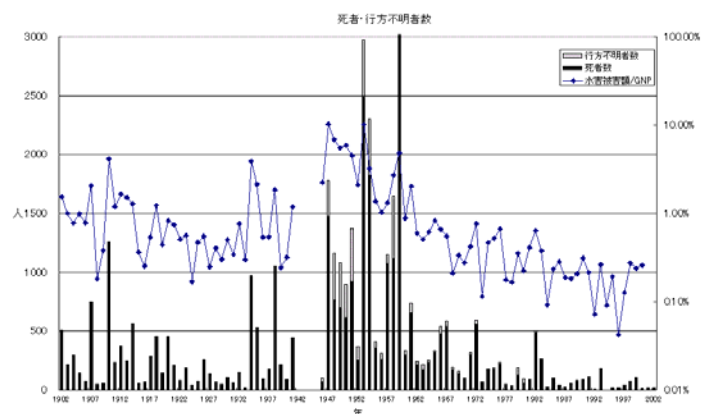
図-3.2.5 我が国の洪水による死者・行方不明者数の推移
