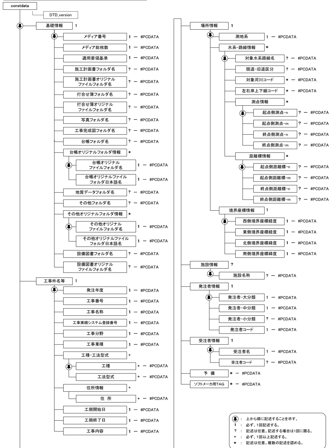
付図 1-1 工事管理ファイルの DTD の構造
