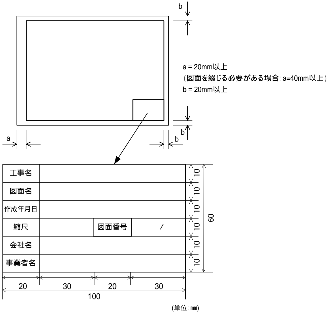
図 5-2 輪郭と余白および表題欄
