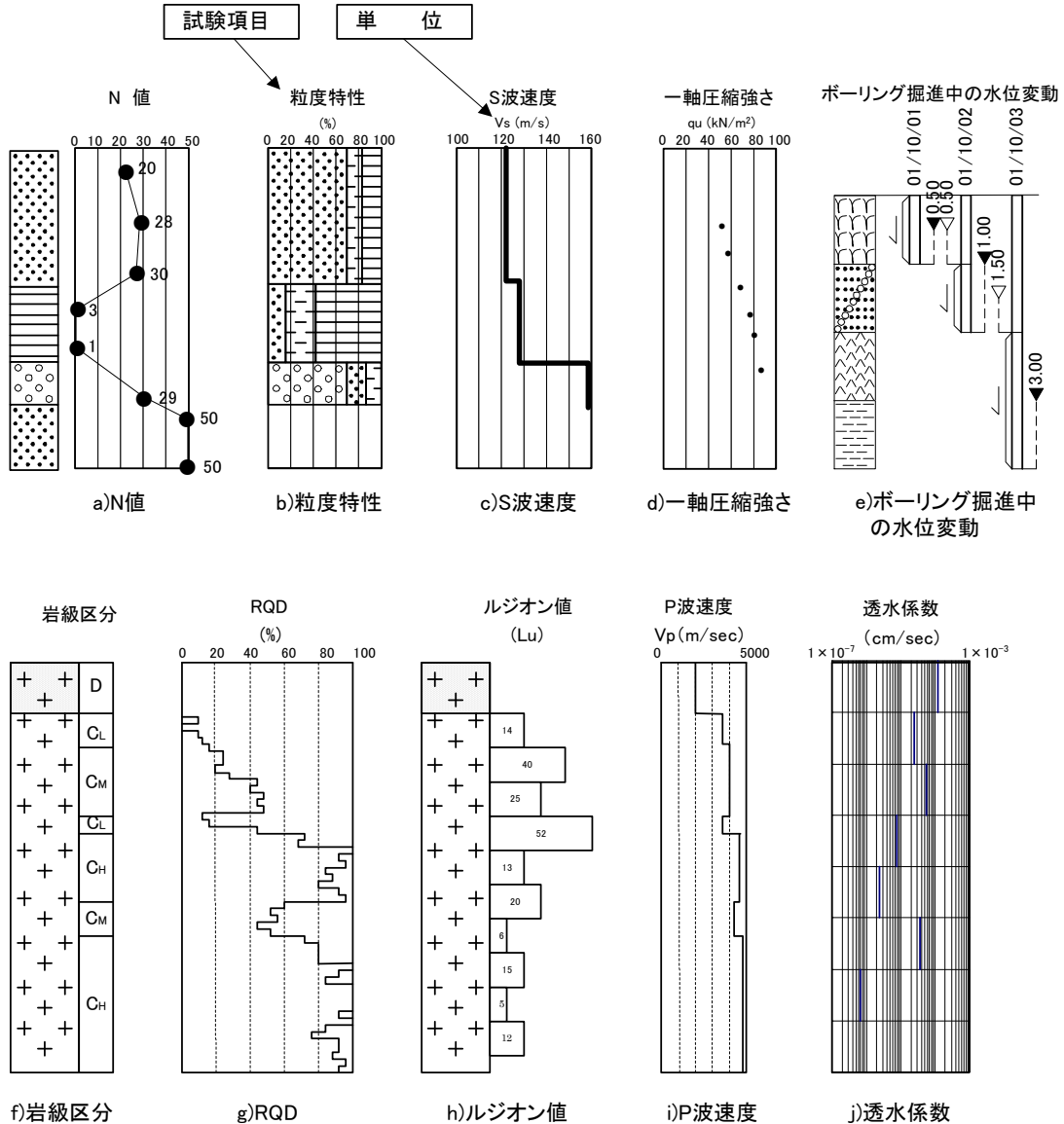
図 3-7 試験・検層データの記載例
