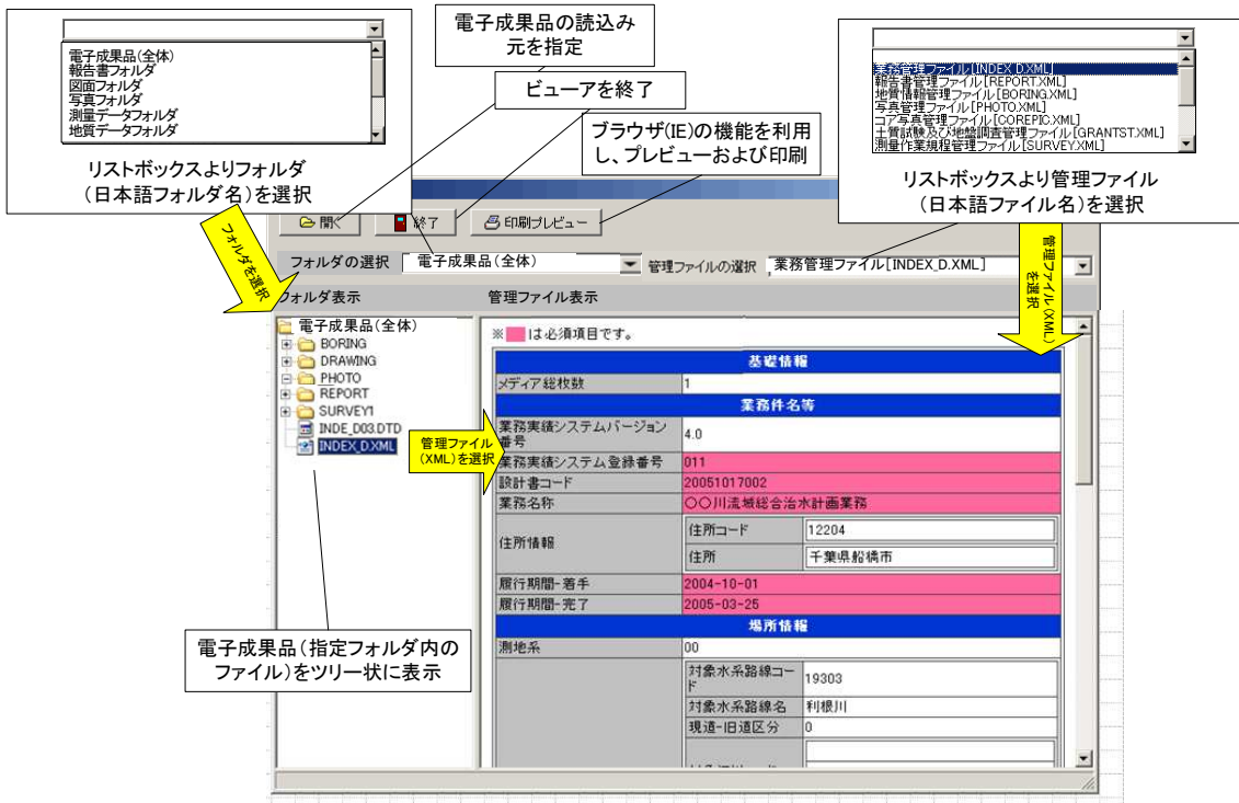
図 1-1 画面イメージ (INDEX_D.XML の例)
