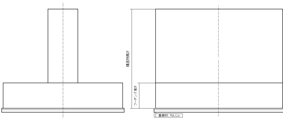
壁式橋脚
