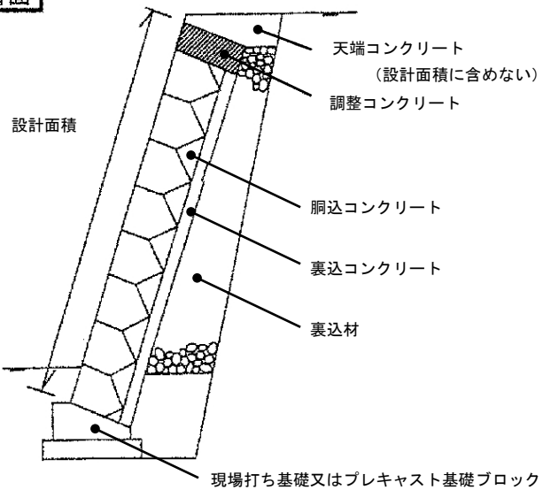
A-A断面
