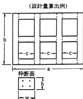
(4本配筋の例)
