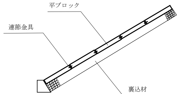
断面図
