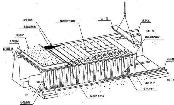
シエツド架設の例 【出典:土木工事標準積算基準書】
